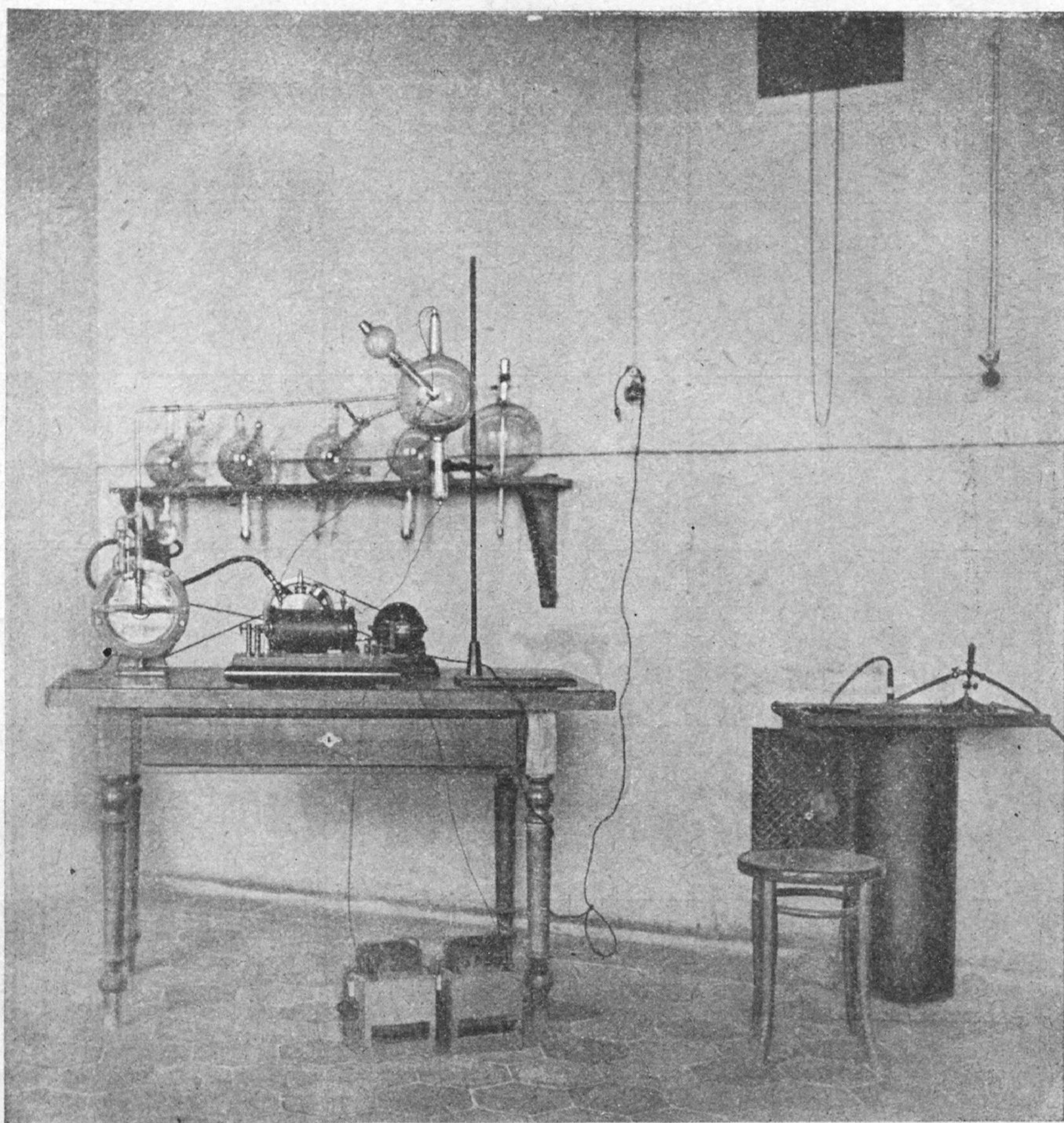
Установка для откачки рентгеновскихъ трубокъ.
