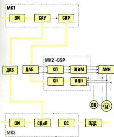
4 Структурная схема МПСУ ЗГПА
