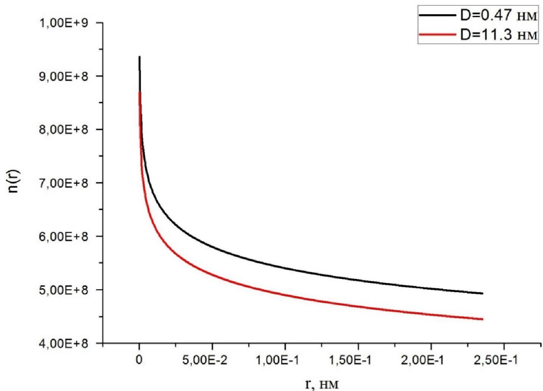
Рисунок 1. Радиальное распределение электронной плотности ОУНТ металлического типа диаметром 0,47 нм и 11,3 нм (armchair – конфигурация)
