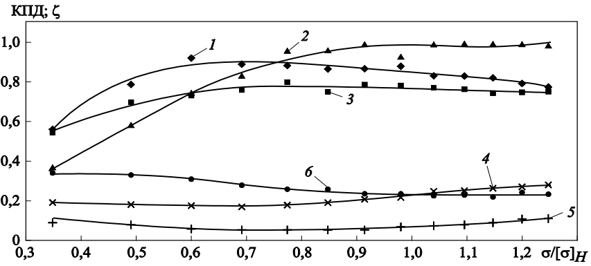
Рис. 6. Зависимость КПД и упругого скольжения при наличии смазочного материала: КПД: 1 — 1 200 об/мин; 2 — 850 об/мин; 3 — 300 об/мин; скольжение: 4 — 1 200 об/мин; 5 — 860 об/мин; 6 — 300 об/мин
