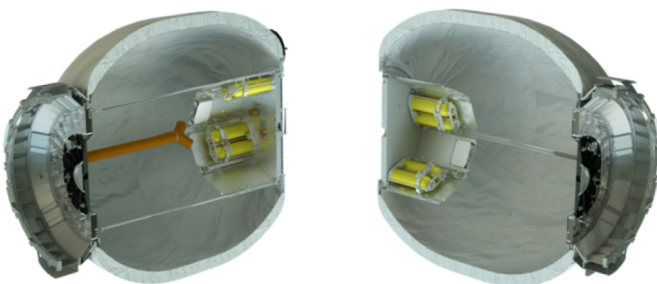
Рис. 2. Одна из концепций компоновки модуля TransHab ( a ) и компоновка экспериментального жилого модуля BEAM ( б ) [24]
