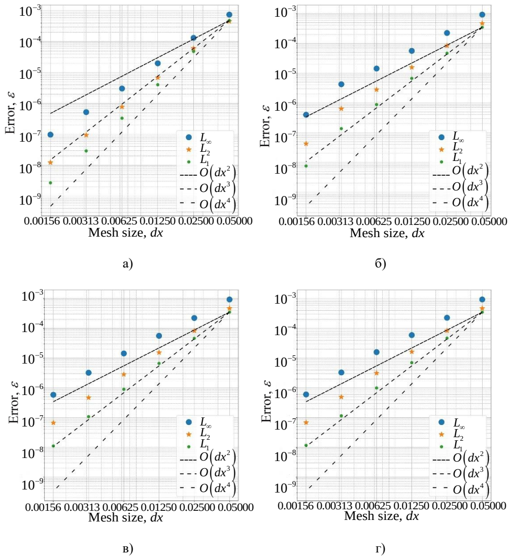
Рис. 1. Логарифмический график ошибки численных методов как функции шага сетки \Delta x для расщеплённого потока Лакса Фридрикса, интегрированного 10-этапным SSP методом Рунге-Кутты 4 порядка с CFL=1, и реконструкциями WENO5-FM (а), WENO9-FM MP (б), WENO9-S MP (в), WENO9-SM MP (г)
