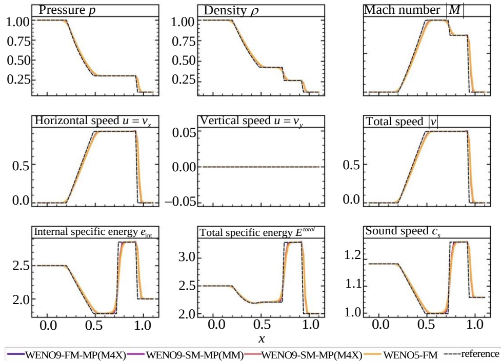
Рис. 2. Профили решения теста Сода вдоль y = 0.5 для потока ЛФ,
