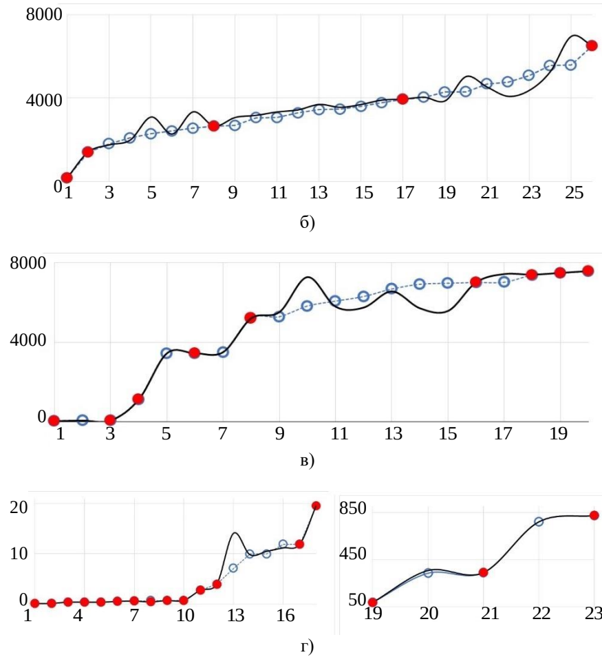
Рис. 4. Результаты тестирования алгоритма идентификации параметров дробно-степенного ряда: а – экспериментальное измерение величины упругого про- скальзывания; б – экспериментальное измерение скорости резания; в – количество деталей в оптимальных партиях обработки; г – годовая технологическая станкоем- кость (результаты, отмеченные красными точками, использовались для идентифи- кации параметров дробно-степенного ряда)
