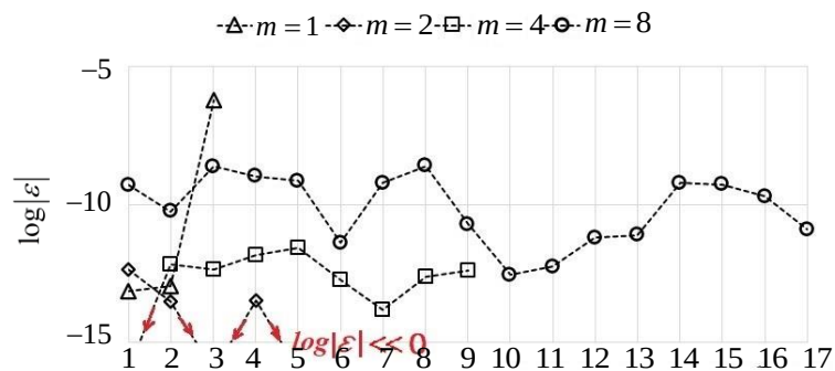
Рис. 5. Относительная погрешность ( \epsilon_i , %) расчета исследуемых откликов в зависимости от размера n матрицы коэффициентов СЛАУ
