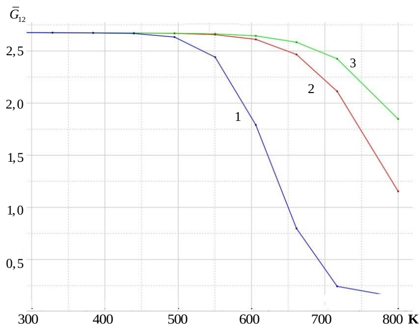
Рис. 9. Изменение эффективного модуля сдвига \bar{G}_{13} тканевого стеклокомпозита в зависимости от температуры нагрева, при разных скоростях нагрева: 1 – 0,8 град/с; 2 – 1,6 град/с; 3 – 4 град/с
