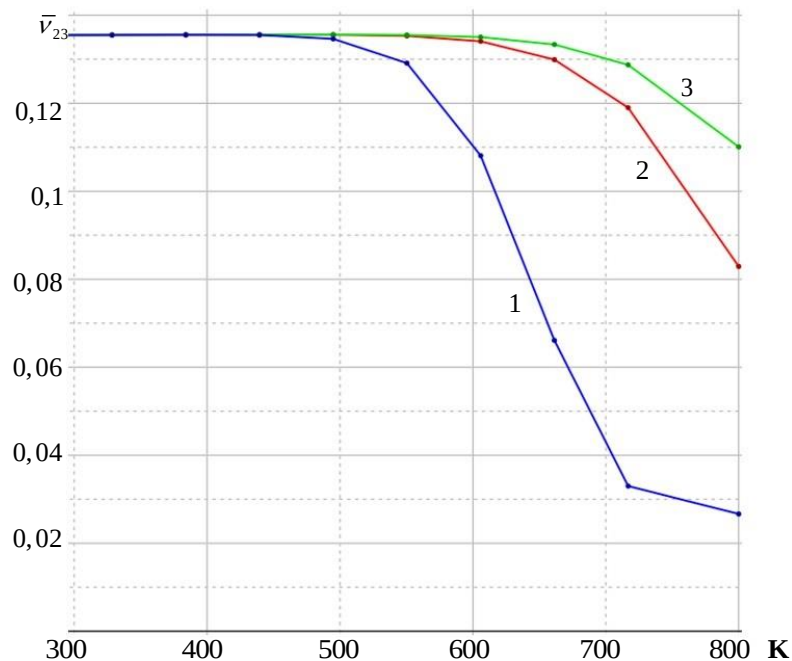
Рис. 8. Изменение эффективного коэффициента Пуассона \bar{\nu}_{23} тканевого стеклокомпозита в зависимости от температуры нагрева, при разных скоростях нагрева: 1 – 0,8 град/с; 2 – 1,6 град/с; 3 – 4 град/с
