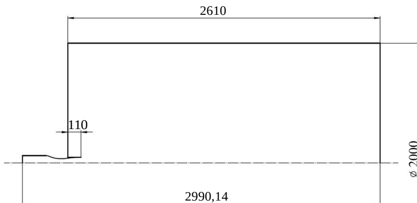
Рис. 2. Габаритные размеры (мм) осесимметричной расчетной области
