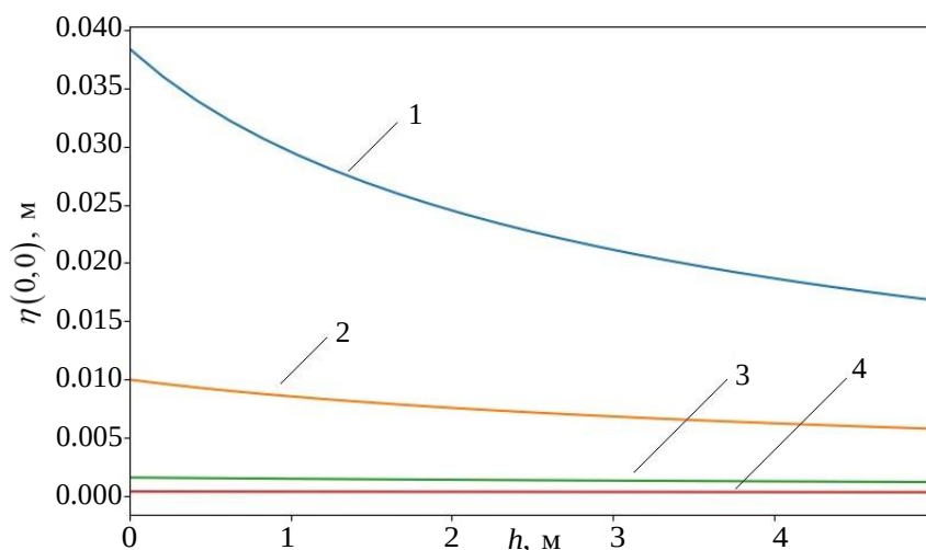
Рис. 5. Зависимость максимального отклонения точки поверхности льда \eta(0,0) (м) от толщины льда h (м) при L = 100 м и различных глубинах источника: 1 — l = 5 м; 2 — l = 10 м; 3 — l = 25 м; 4 — l = 50 м
