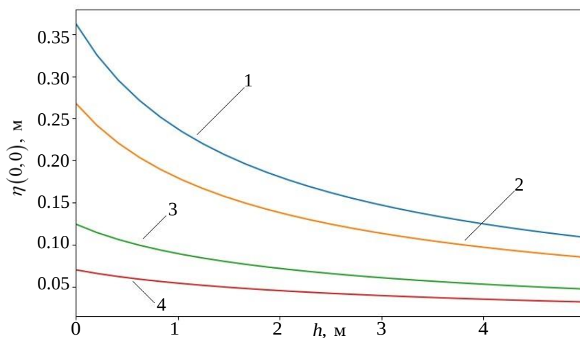
Рис. 4. Зависимость максимального отклонения точки поверхности льда \eta(0,0) (м) от толщины льда h (м) при L = 5 м и различных глубинах источника: 1 — l = 0,5 м; 2 — l = 1 м; 3 — l = 2,5 м; 4 — l = 5 м
