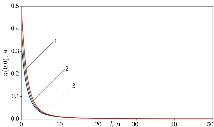
Рис. 7. Зависимость максимального отклонения точки поверхности льда \eta(0,0) (м) от глубины источника l (м) при различных толщинах льда: 1 — h = 1 м; 2 — h = 0,5 м; 3 — h = 0,1 м
