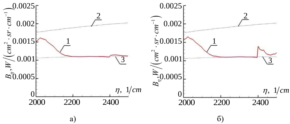
Рис. 6. Функция Планка в слое газа CO 2 в области 4.3 мкм. Анализ воздействия неравновесности по температуре ассиметричной колебательной моды. T_{v1} = T_{v2} = 1250K, T = T_{v3} = T_r = 1550K .
