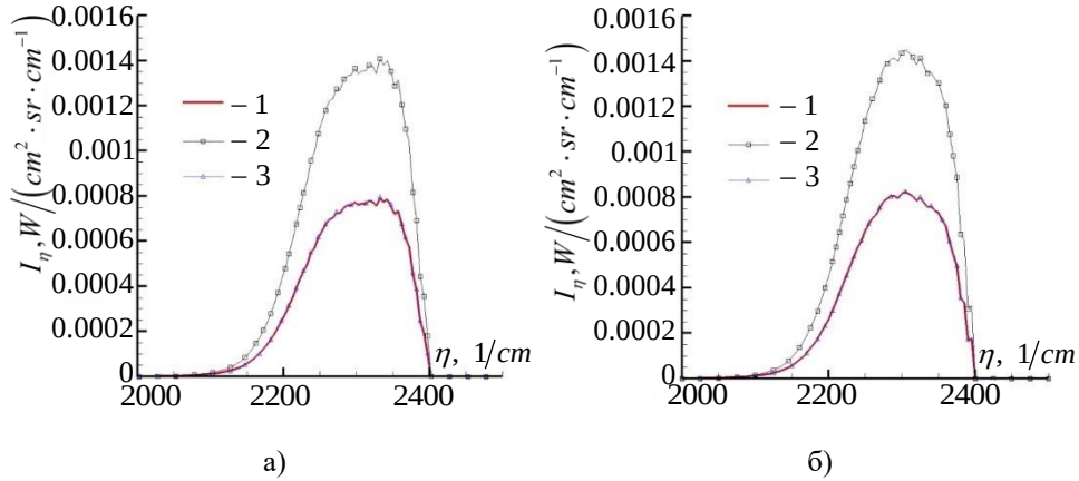
Рис. 5. Яркость слоя газа CO 2 в области 4.3 мкм. Анализ воздействия неравновесности по температуре ассиметричной колебательной моды.
