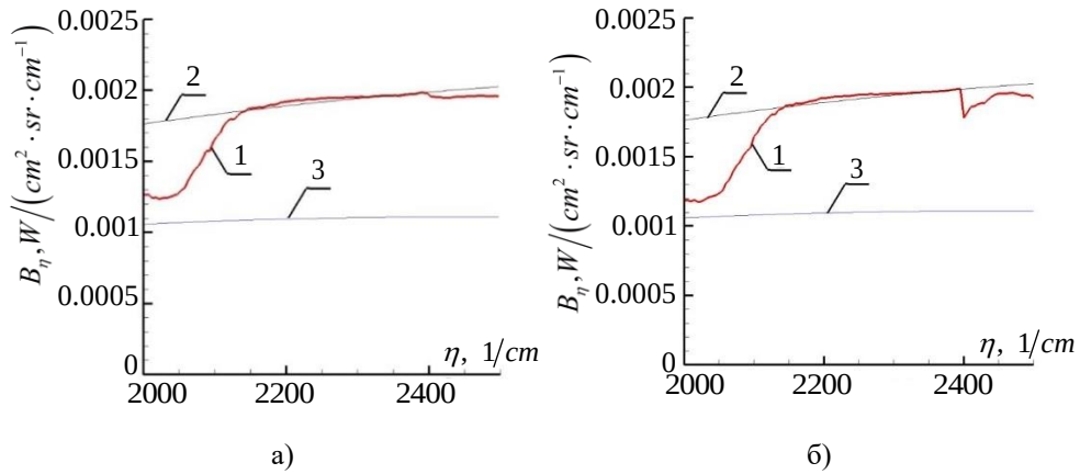
Рис. 3. Функция Планка в слое газа \text{CO}_2 в области 4.3 мкм. Анализ воздействия неравновесности по температуре деформационной колебательной моды. T_{v1} = T_{v2} = 1250\text{K} , T = T_{v3} = T_r = 1550\text{K} .
