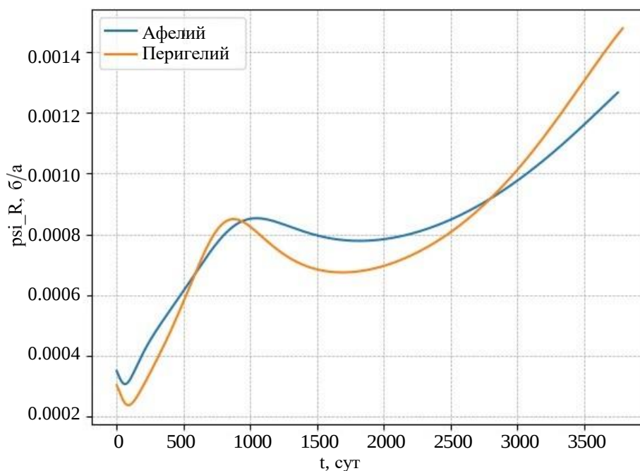
Рис. 8. Сравнение зависимостей сопряженной переменной \psi_R от времени при крайних условиях орбиты Юпитера в афелии и перигелии
