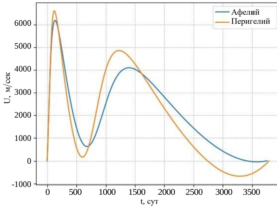
Рис. 4. Сравнение зависимостей радиальной скорости КА U от времени при крайних условиях орбиты Юпитера в афелии и перигелии
