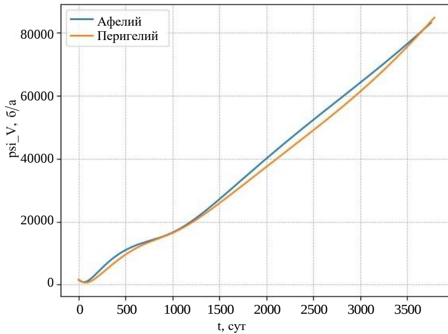
Рис. 10. Сравнение зависимостей сопряженной переменной \psi_v от времени при краевых условиях орбиты Юпитера в афелии и перигелии
