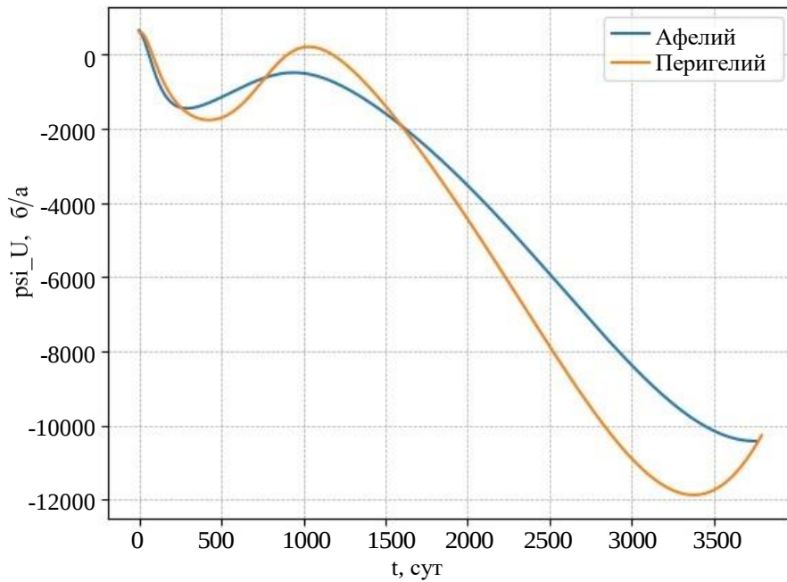
Рис. 9. Сравнение зависимостей сопряженной переменной \psi_u от времени при краевых условиях орбиты Юпитера в афелии и перигелии
