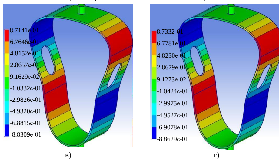
Рис. 6. Поля компоненты \omega_1 , отвечающие второй собственной форме потери устойчивости композитной конструкции для различных моментов времени ее отверждения: а — 1 740; б — 5 220 с; в — 15 660 с; г — 17 400 с
