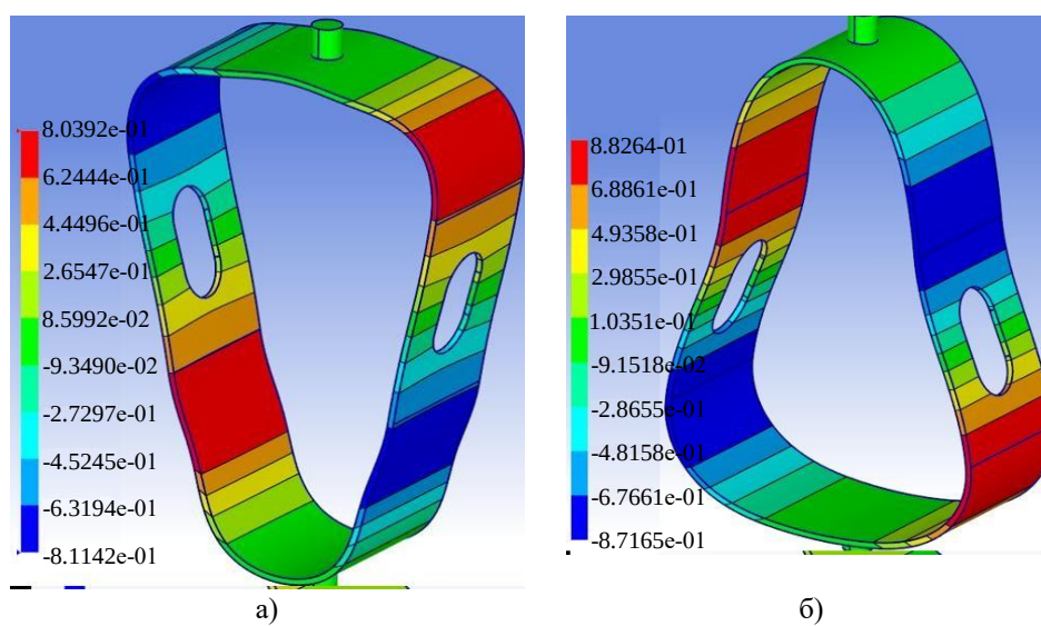
Рис. 5. Поля компоненты \omega_1 , отвечающие первой собственной форме потери устойчивости композитной конструкции для различных моментов времени ее отверждения: а — 1 740; б — 5 220 с; в — 15 660 с; г — 17 400 с
