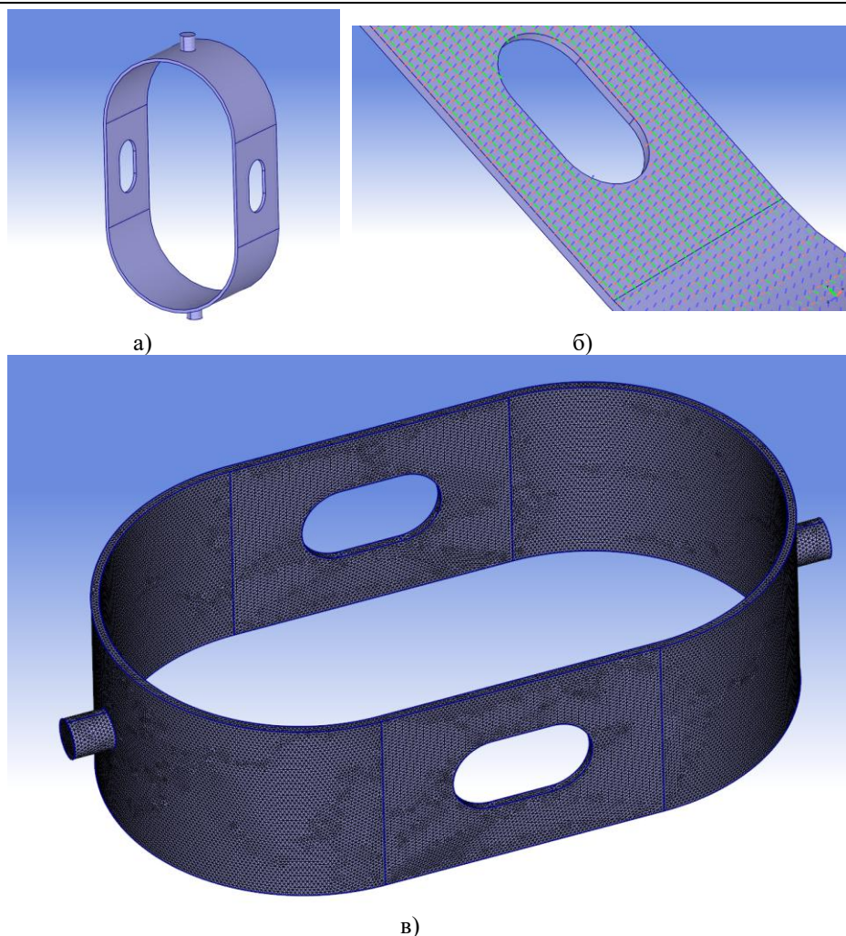
Рис. 1. Модель композитного элемента конструкции, для которого проводилось численное моделирование: а — общий вид; б — локальные базисы криволинейной ортотропии; в — конечно-элементная сетка
