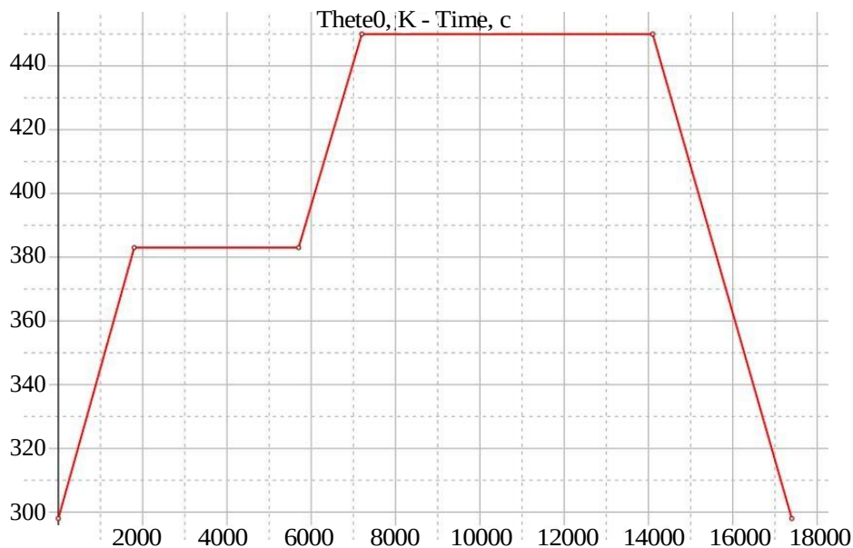
Рис. 2. График изменения температуры внешней среды \theta_e(t)
