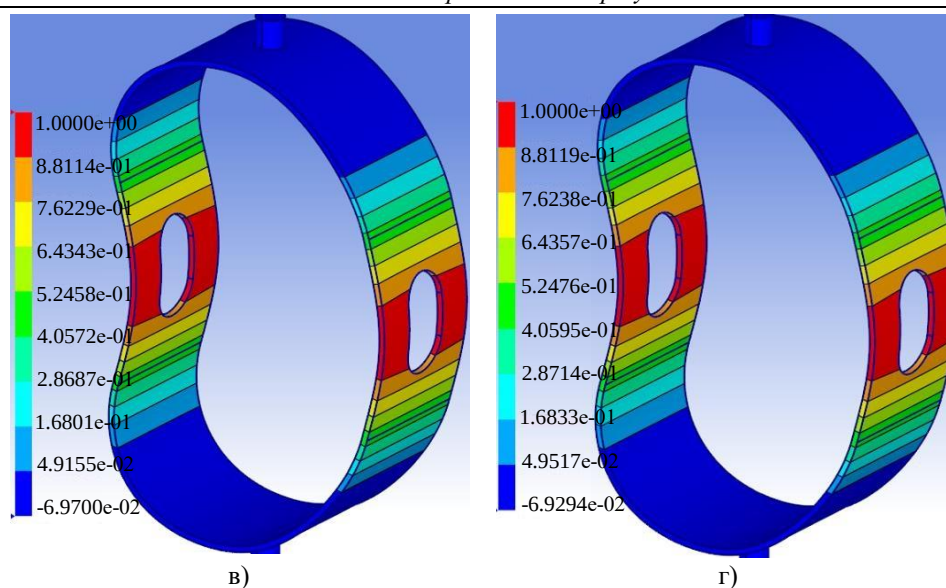
Рис. 7. Поля компоненты \omega_1 , отвечающие третьей собственной форме потери устойчивости композитной конструкции для различных моментов времени ее отверждения: а — 1 740; б — 5 220 с; в — 15 660 с; г — 17 400 с
