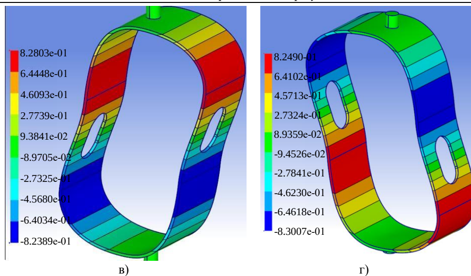
Рис. 5. Поля компоненты \omega_1 , отвечающие первой собственной форме потери устойчивости композитной конструкции для различных моментов времени ее отверждения: а — 1 740; б — 5 220 с; в — 15 660 с; г — 17 400 с
