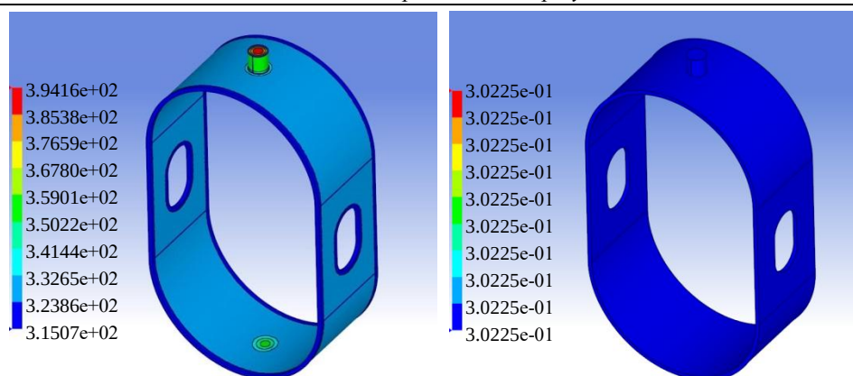
Рис. 2. Распределения температуры (слева) и объемной концентрации твердого полимера (справа), полученные в результате решения задачи отверждения: а — 3 480 с; б — 5 220 с; в — 13 920 с; г — 17 400 с
