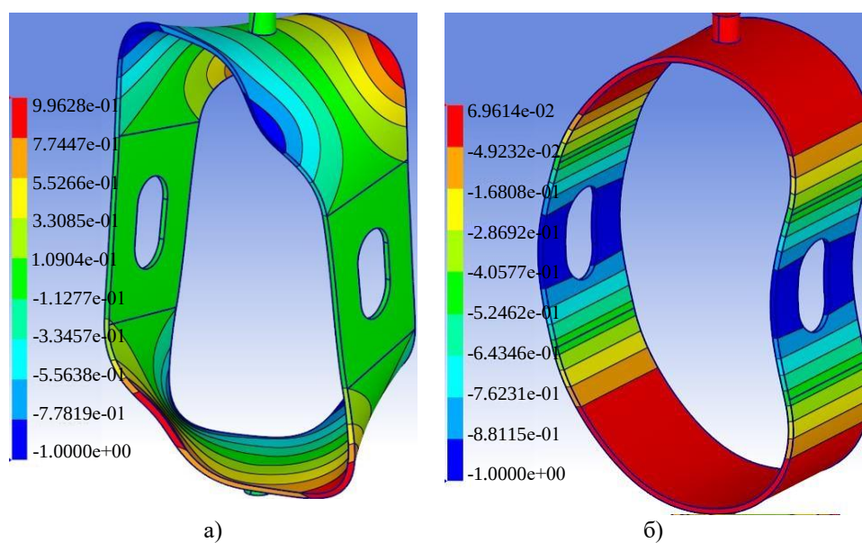
Рис. 6. Поля компоненты \omega_1 , отвечающие второй собственной форме потери устойчивости композитной конструкции для различных моментов времени ее отверждения: а — 1 740; б — 5 220 с; в — 15 660 с; г — 17 400 с
