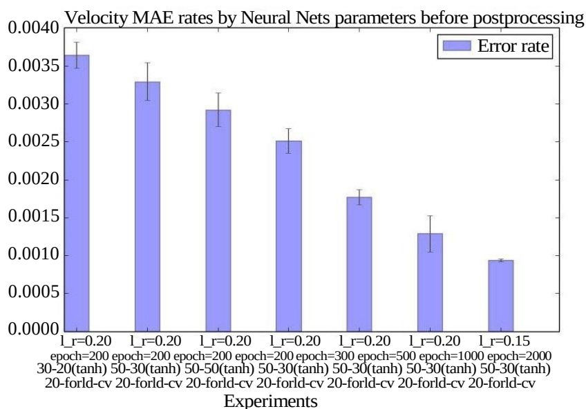
Рис. 4. Значения среднемодульных отклонений и их дисперсий, l_r — скорость обучения, k - fold - cv — кроссвалидация по k блокам, epoch — количество эпох, t - n ( \tanh ) — m нейронов на первом скрытом слое, n — нейронов на втором скрытом слое с функцией активации гиперболический тангенс
