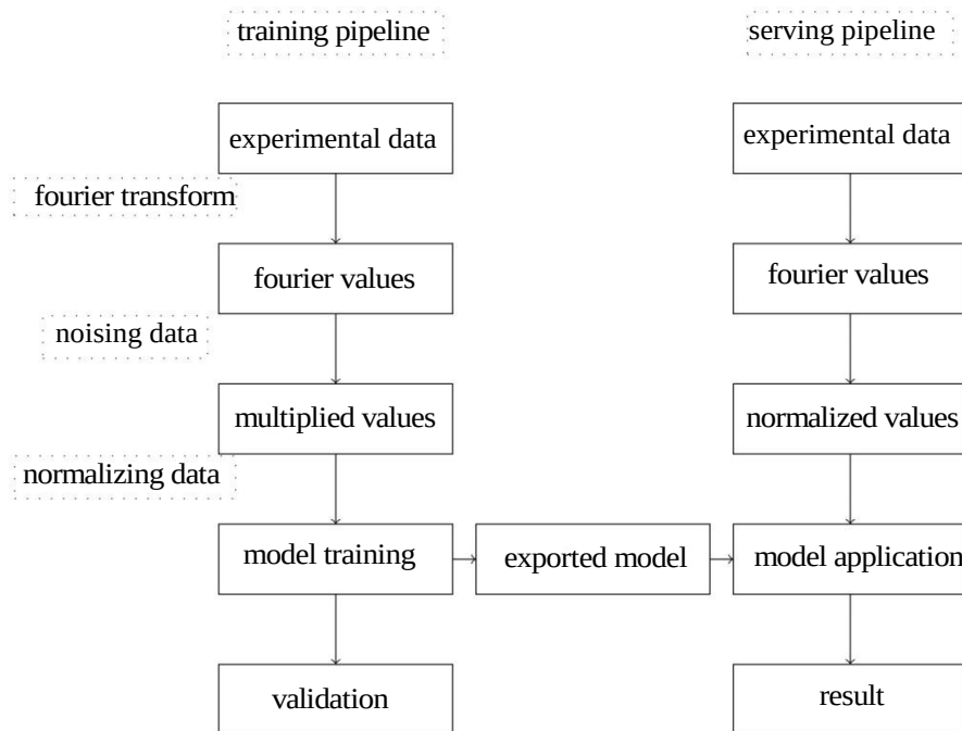
Рис. 9. Структурная схема разработанного алгоритма обучения нейронной сети для предсказания глубины и скорости
