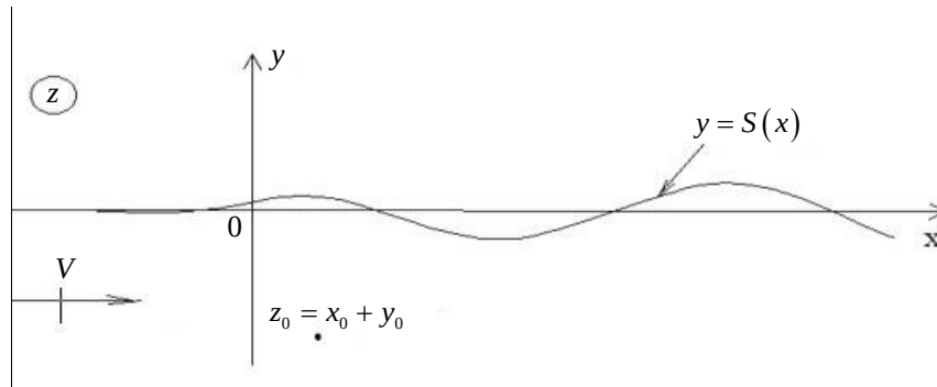
Рис. 1. Общая схема обтекания точечной гидродинамической особенности потоком со свободной границей
