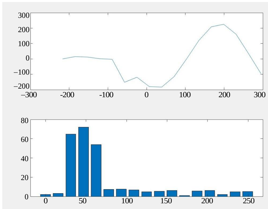
Рис. 3. Тангенс угла наклона волны поверхностного возмущения и её спектр, полученный методом быстрого преобразования Фурье
