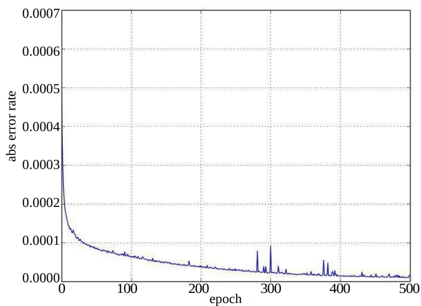
Рис. 8. График зависимости среднего модуля отклонения скорости прохождения цилиндра до постпроцессинга от количества эпох: epoch — количество эпох обучения перед валидационной оценкой,
