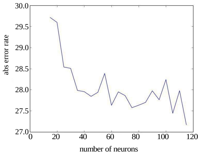
Рис. 6. График зависимости среднего модуля отклонения до постпроцессинга от количества нейронов в скрытом слое однослойной нейронной сети: numbers of neurons – количество нейронов,
