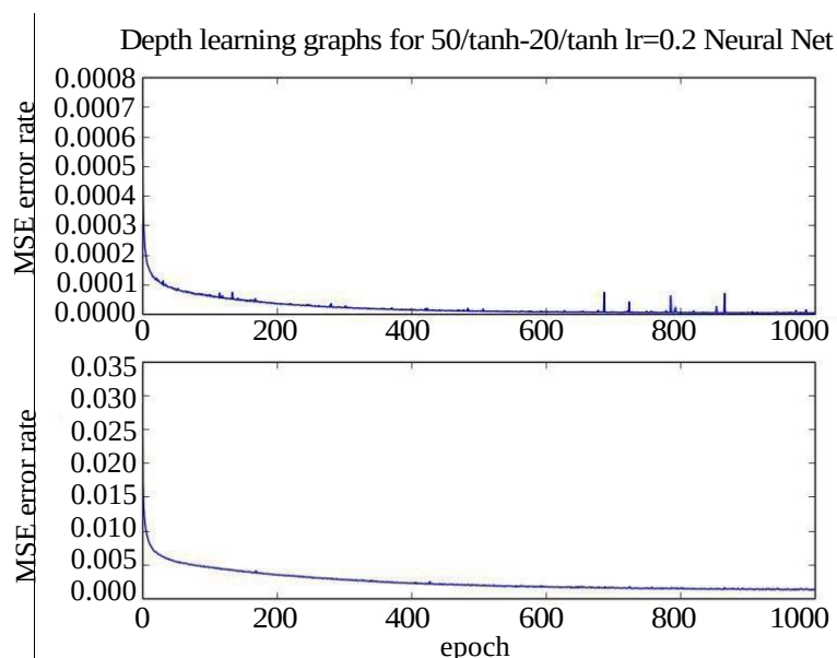
Рис. 5. Графики зависимостей MSE, MAE от количества эпох соответственно
