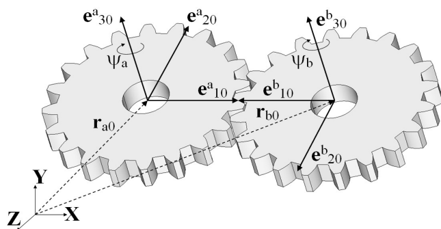
Рис. 1. Исходное положение зубчатой передачи
