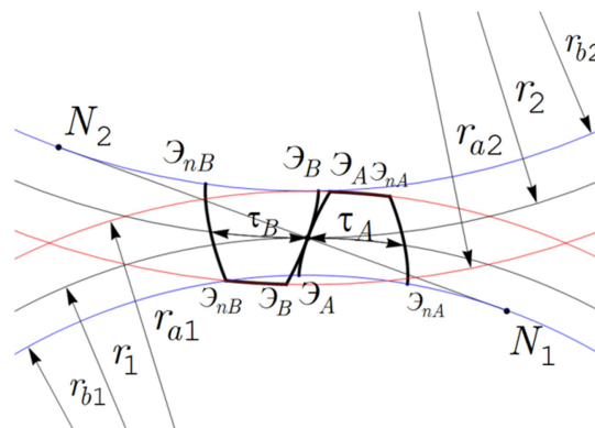
Рис. 3. Прямозубое эвольвентное зацепление Эвольвентный профиль \mathcal{E}_A \mathcal{E}_A колеса A описывается через
