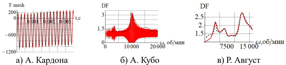
Рис. 2. Результаты сравнения верификационных тестов, полученных с помощью авторской модели (красный) с результатами других авторов (черный)
