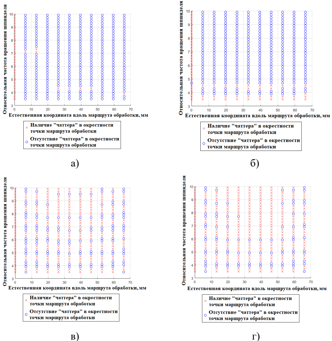
Рис. 9. Расчетные карты виброустойчивости процесса фрезерования вдоль траектории маршрута обработки для различных значений заднего угла режущего клина концевой фрезы: а) \gamma = 1^\circ ; б) \gamma = 3^\circ ; в) \gamma = 5^\circ ; г) без учета сил контактного взаимодействия по задней поверхности фрезы
