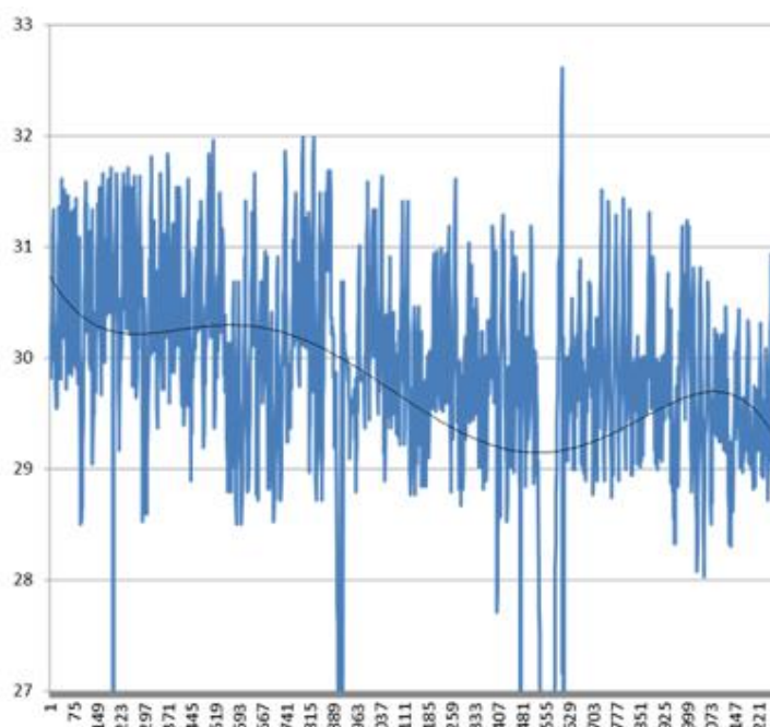
Рис. 6 Тренд изменения напряжения АБ
