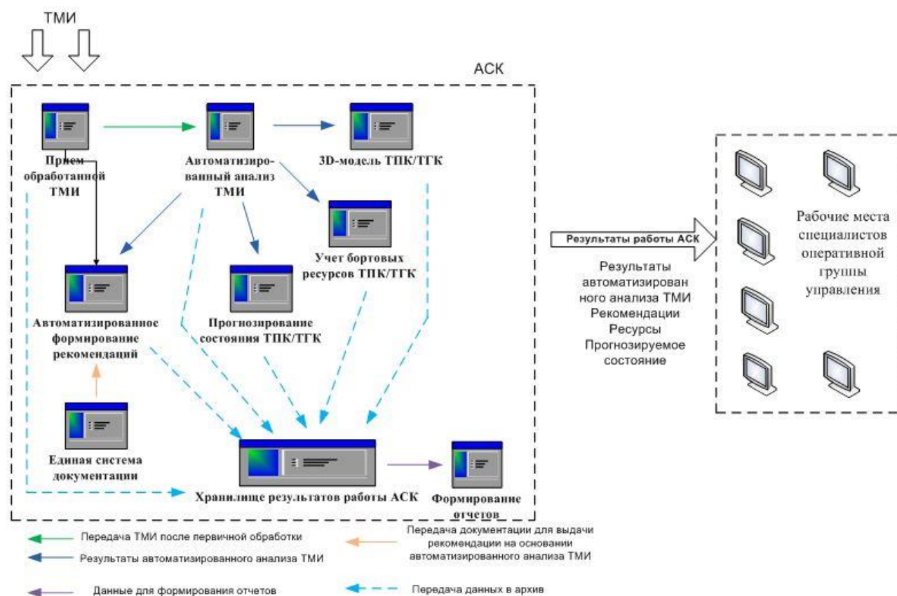
Рис. 9. Функциональная схема АСК.
