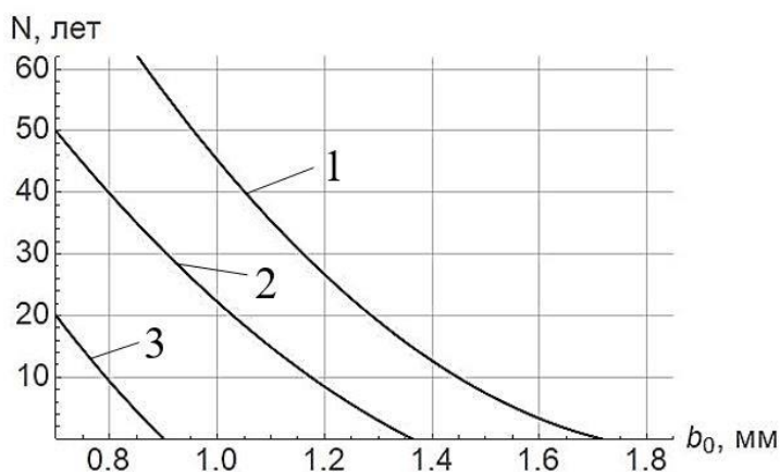
Рис. 11. Зависимость ресурса от начальной глубины трещины для соотношений полудлины и глубины: b/a = 2 (1), b/a = 1 (2), b/a = 1/2 (3)
