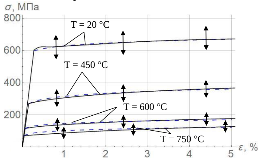
Рис. 1. Кривые растяжения феррито-перлита: эксперимент (сплошные линии), расчет (синие пунктирные линии)
