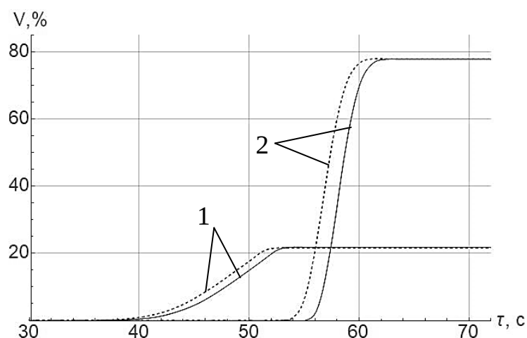
Рис. 5. Распределение удельных долей в окрестности сварного шва: поверхностный слой (штриховые линии), срединный слой (сплошные линии)
