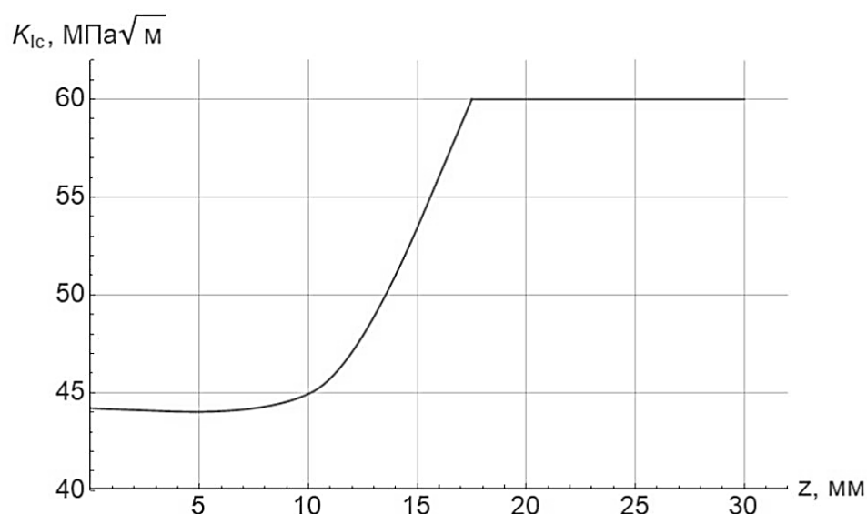
Рис. 7. Вязкость разрушения гетерогенной структуры
