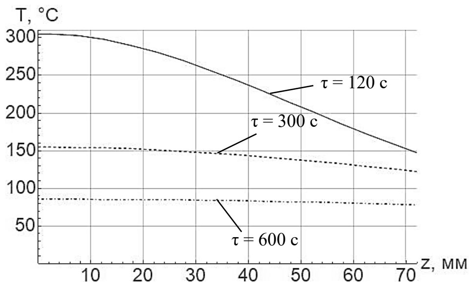
Рис. 4. Распределение температур по длине
