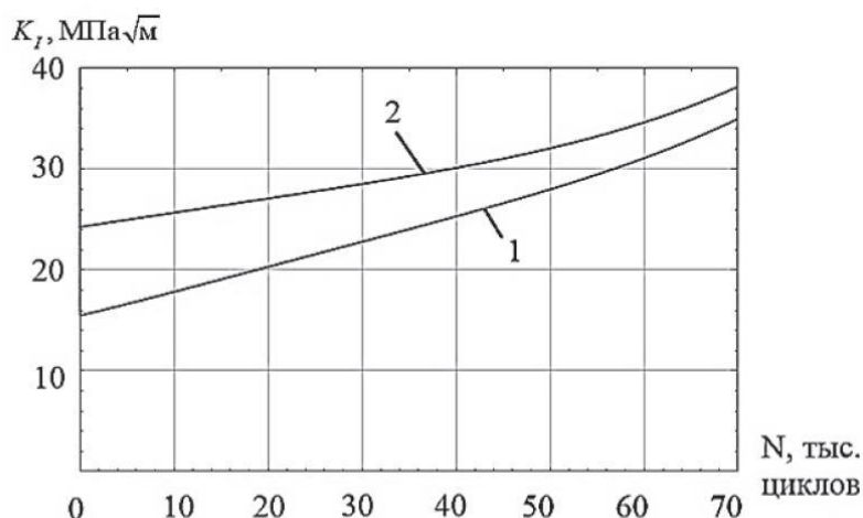
Рис. 10. Изменение КИН в наиболее заглубленной точке (1) и точке, выходящей на поверхность (2) для трещины с начальными размерами b_0 = 1 мм, a_0 = 0,5 мм
