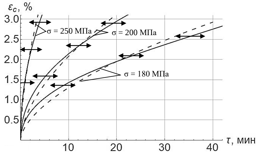
Рис. 2. Кривые ползучести феррито-перлита при T = 500^\circ\text{C} : эксперимент (сплошная линия), расчет (пунктирная линия)
