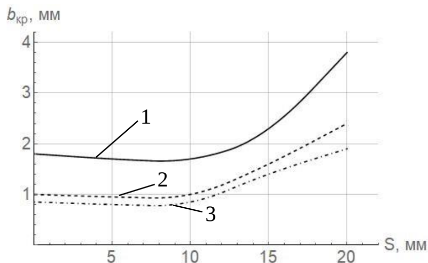
Рис. 8. Зависимость критической глубины от расстояния до центра сварного шва: a/b=1 (1), a/b=3 (2), a/b=5 (3)
