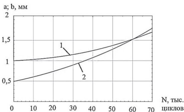
Рис. 9. Изменение глубины (1) и полудлины (2) для трещины с начальными размерами b_0=1 мм, a_0=0,5 мм
