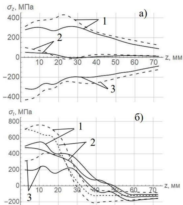
Рис. 6. Распределение осевых (а) и окружных (б) остаточных сварочных напряжений по длине трубы для: 1 – внутренней, 2 – срединной, 3 – внешней поверхностей для упруговязкопластического (сплошные линии) и упругопластического (штриховые линии) решения
