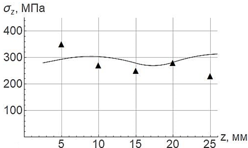
Рис. 3. Распределение по длине осевых остаточных сварочных напряжений на внутренней поверхности трубы: сплошная линия – расчет, маркеры – эксперимент
