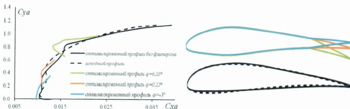
Рис. 10 Сравнение результатов оптимизации профилей крыла
