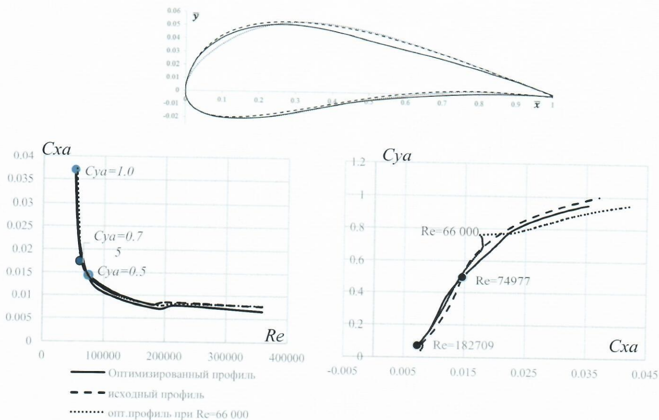
Рис. 11 Сравнение аэродинамических характеристик исходного и оптимизированного профилей
