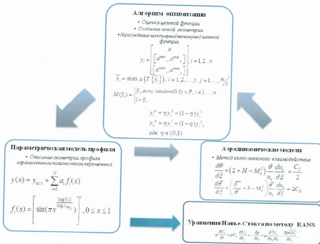
Рис. 1. Блок-схема прямого метода численной оптимизации
