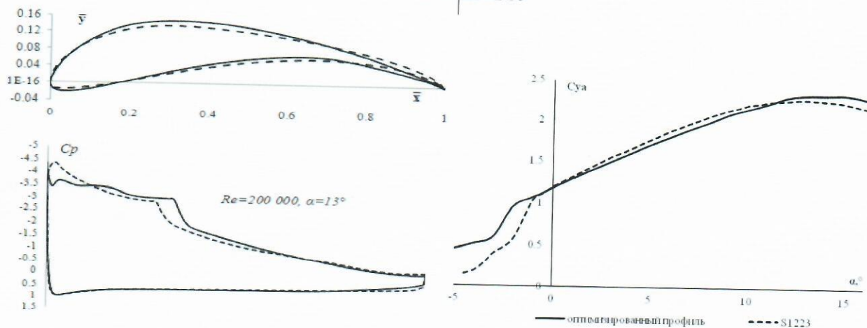
Рис. 3 Сравнение контуров и аэродинамических характеристик исходного и оптимизированного профилей по критерию увеличения коэффициента подъемной силы
