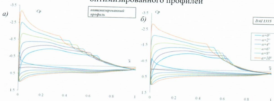
Рис. 8. Сравнение распределений давлений исходного(б) и оптимизированного(а) профилей при различных углах атаки
