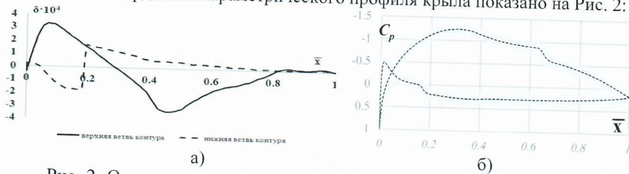
Рис. 2. Оценка точности аппроксимации параметрического контура: а) оценка отклонения ординат исходного контура от аппроксимированного; б) сравнение распределений давления исходного аппроксимируемого контуров
