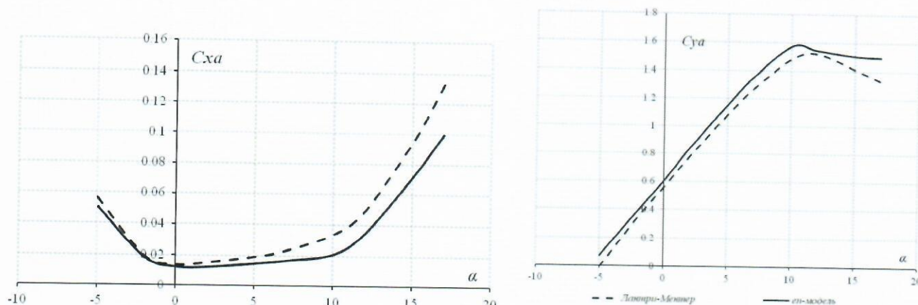
Рис. 9. Сравнение аэродинамических характеристик профиля крыла при использовании различных аэродинамических моделей
