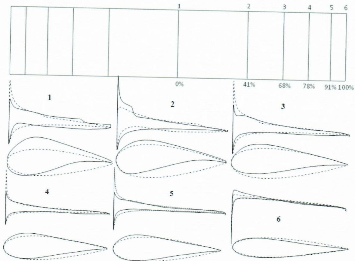
Рис. 13. Сравнение распределений давления по сечениям исходного (пунктирная линия) и оптимизированного (сплошная линия) крыльев
