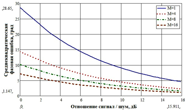
Рисунок 12. Фазовая ошибка калибровки
