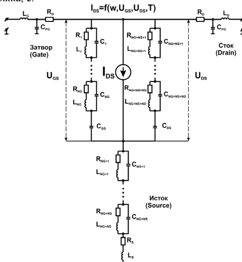
Рисунок 10. Эквивалентная электрическая схема мощного АЭ на плате
