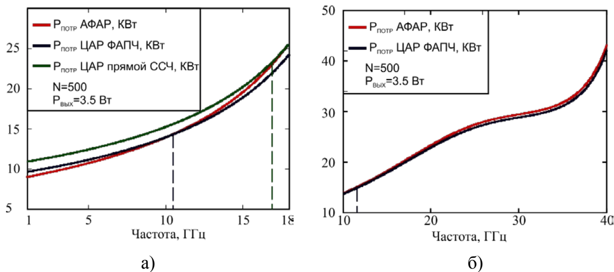
Рисунок 3. Потребляемые мощности АФАР и ЦАР
