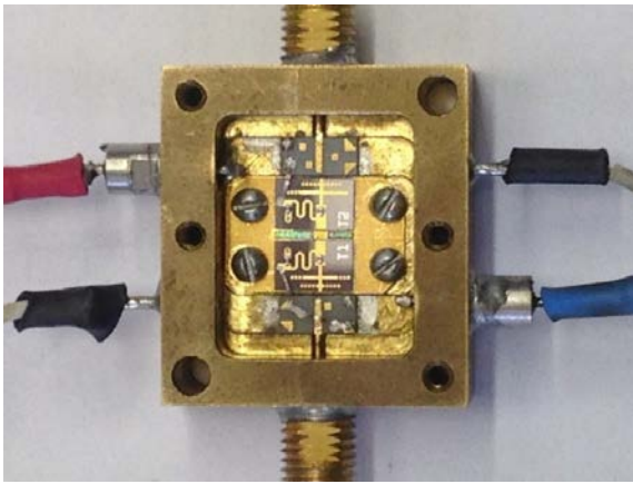
Рисунок 15. АЭП в корпусе
