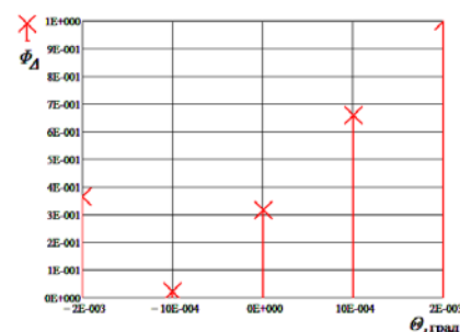
Рисунок 25. Разностная ДН экспериментальной ЦАР, шаг выборки 0,01 град.
