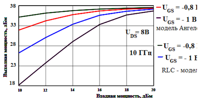
Рисунок 19. Сравнение выходной мощности
