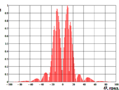
Рисунок 24. Разностная ДН экспериментальной ЦАР, угол прихода 0 град.
