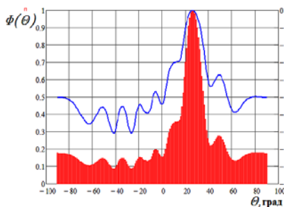
Рисунок 26. ДН экспериментальной ЦАР, угол прихода 26 град.
