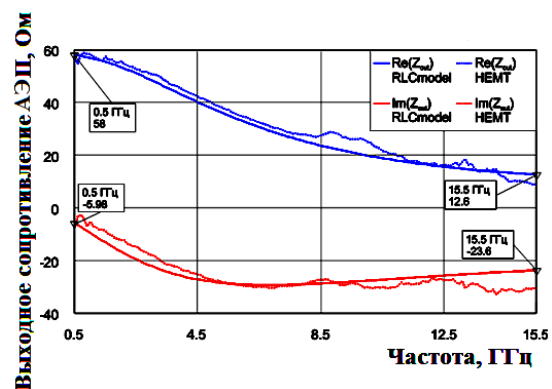
Рисунок 18. Верификация выходного сопротивления АЭП
