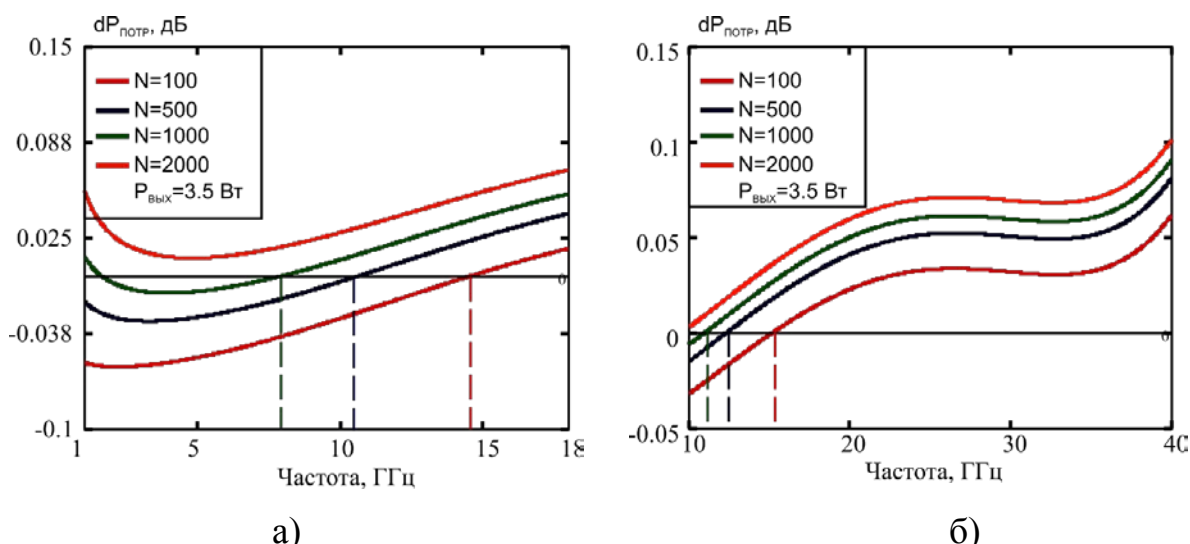
Рисунок 5. Частотная зависимость dP_{\text{потр}} при различных значениях N
