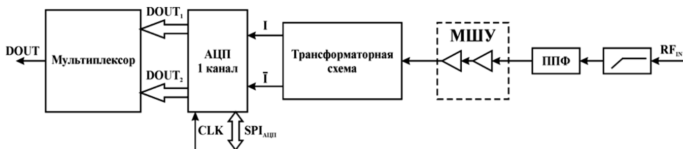
Рисунок 8. Структурная схема приёмного тракта ЦППМ с преобразованием на несущей при использовании трансформаторной схемы
