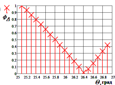
Рисунок 27. Разностная ДН экспериментальной ЦАР, шаг выборки 0,1 град. угол прихода 26,4 град.
