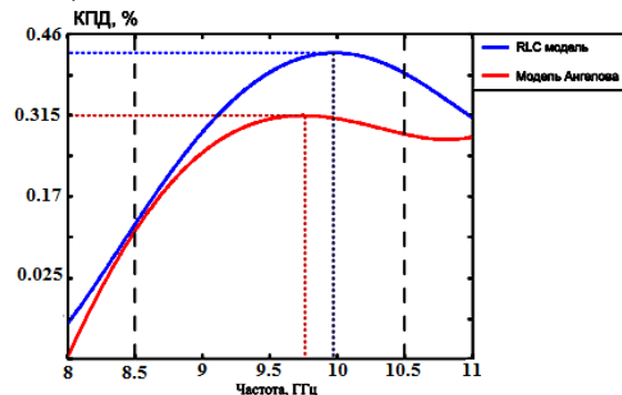
Рисунок 20. Сравнение КПД СВЧ УМ
