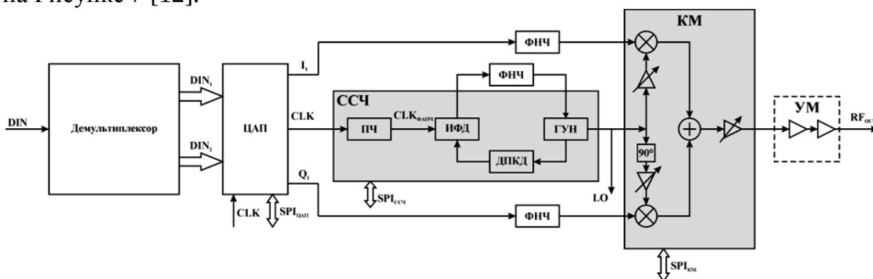
Рисунок 7. Структурная схема передающего тракта модуля ЦАР с ССЧ на основе цифрового кольца ФАПЧ
