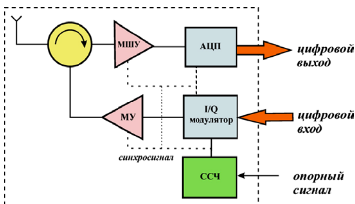
Рисунок 6. Структурная схема модуля ЦАР
