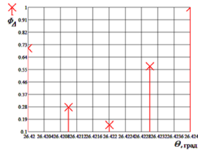
Рисунок 28. Разностная ДН экспериментальной ЦАР, шаг выборки 0,001 град. угол прихода 26,422 град.
