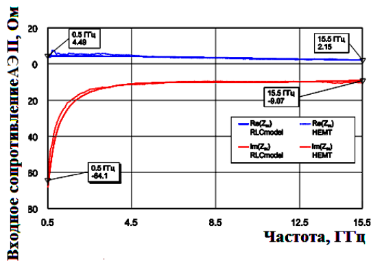
Рисунок 17. Верификация входного сопротивления АЭП
