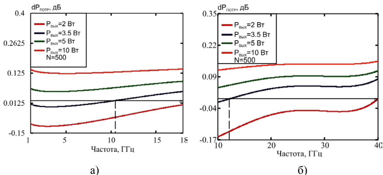
Рисунок 4. Частотная зависимость dP_{\text{потр}} при различных значениях P_{\text{вых}}
