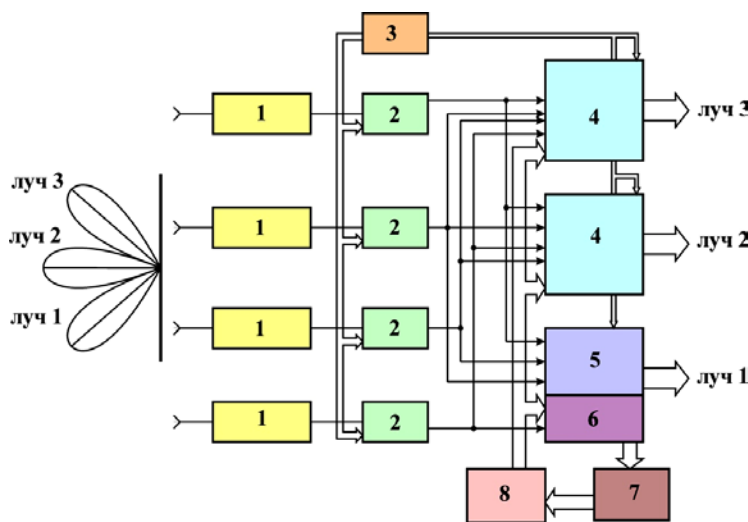
Рисунок 11. Устройство калибровки ЦАР составе блока калибровки; 8 – блок расчета амплитудных и фазовых коэффициентов в составе блока калибровки.
