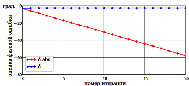
Рисунок 29. Сходимость процесса калибровки экспериментальной ЦАР
