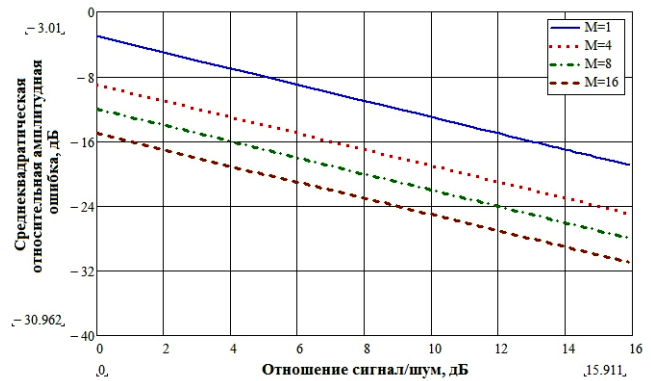
Рисунок 13. Относительная амплитудная ошибка калибровки
