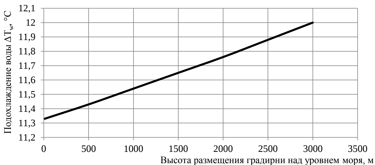
Рисунок 7. Зависимость показателя глубины подохлаждения воды в градирни от высоты размещения над уровнем моря.
