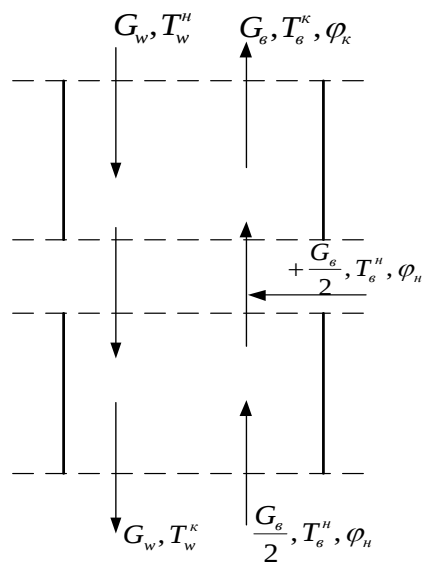
Рисунок 5. Схема расчета градирни с промежуточной подачей воздуха
