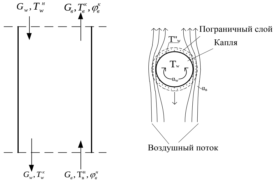
Рисунок 1. Схема взаимодействия между охлаждаемой водой и воздухом.
