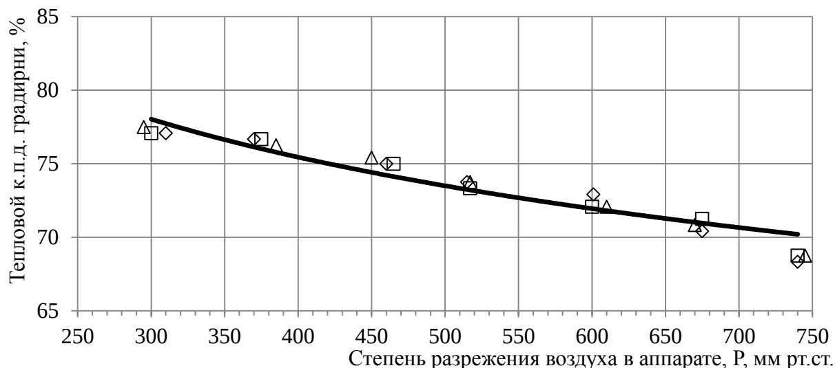
Рисунок 12. График зависимости теплового к.п.д. градирни от степени разрежения воздуха в аппарате.
