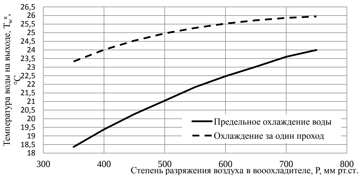
Рисунок 6. График зависимости конечной температуры воды на выходе из водоохладителя от степени разрежения воздуха.
