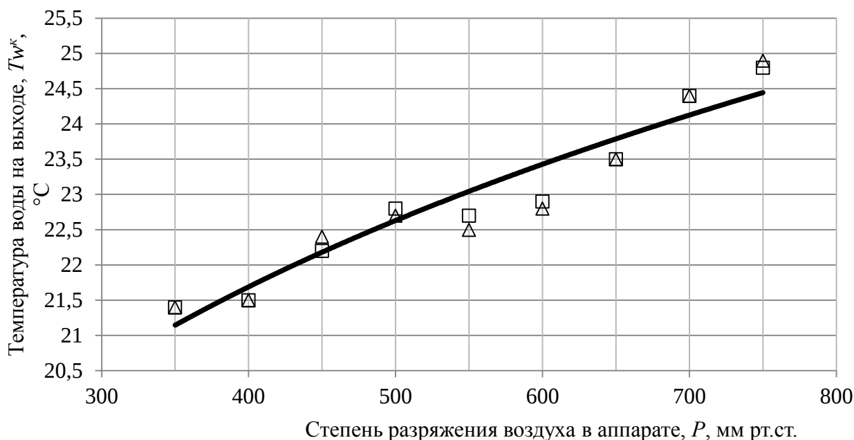
Рисунок 10. График зависимости предельно достижимой температуры воды от степени разряжения воздуха.
