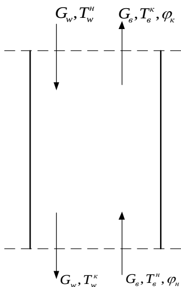
Рисунок 4. Схема расчета градирни с одиночной подачей воздуха
