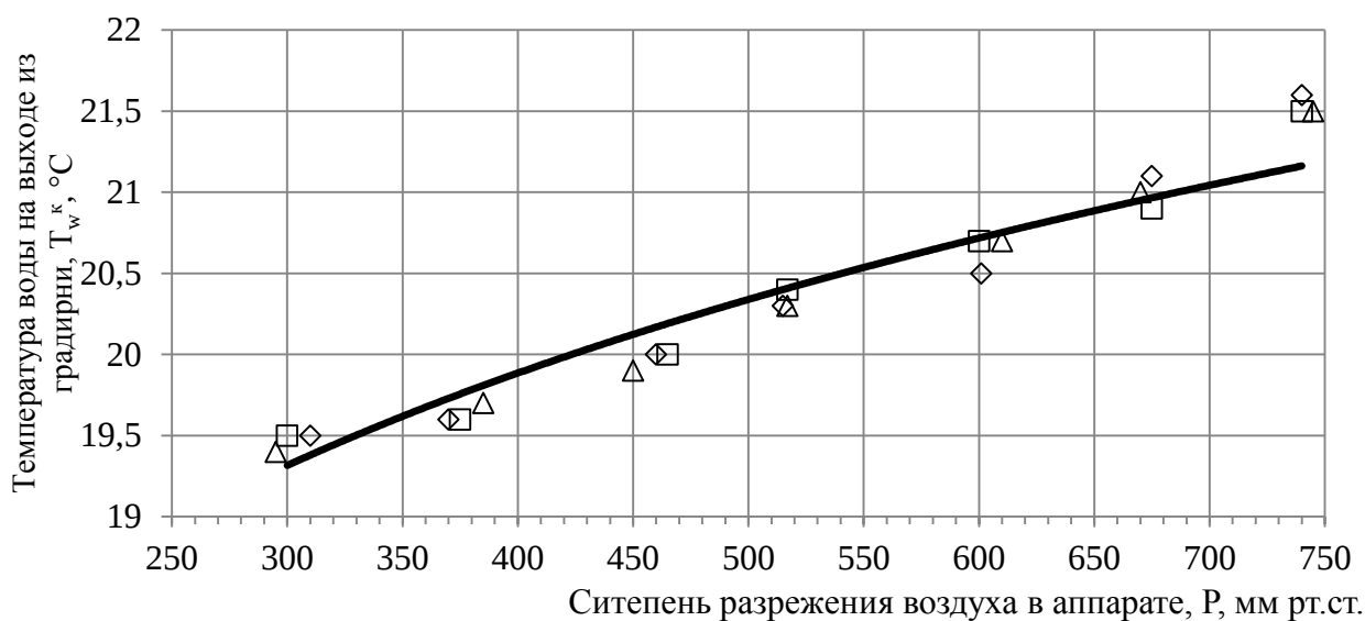
Рисунок 11. График зависимости температуры воды на выходе из градирни от степени разряжения воздуха.
