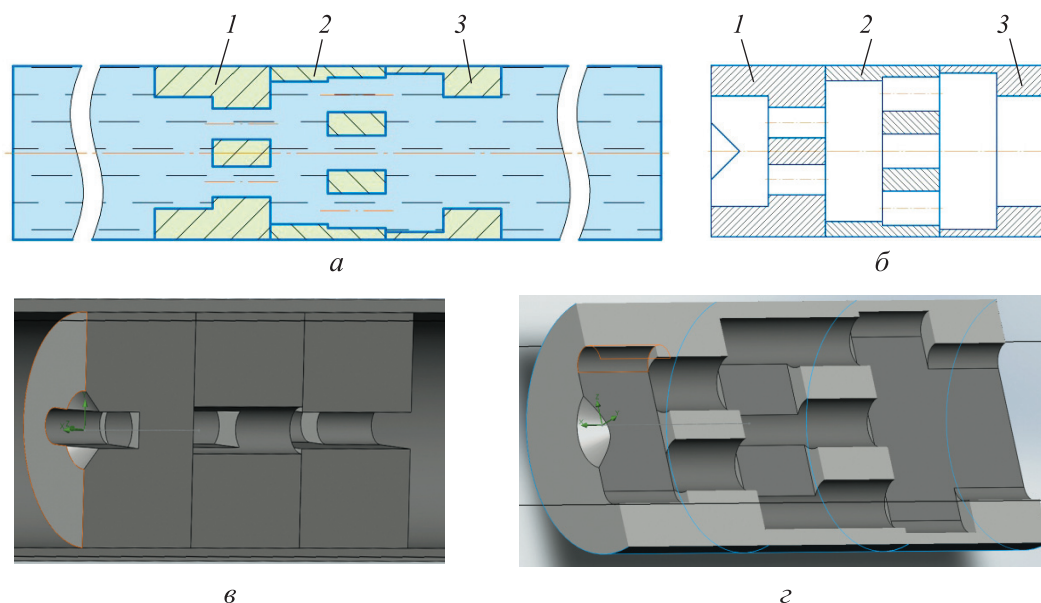
Рис. 2. Схемы расчета (а), разреза (б), поперечного (в) и продольного разрезов (г) третьего канала:
