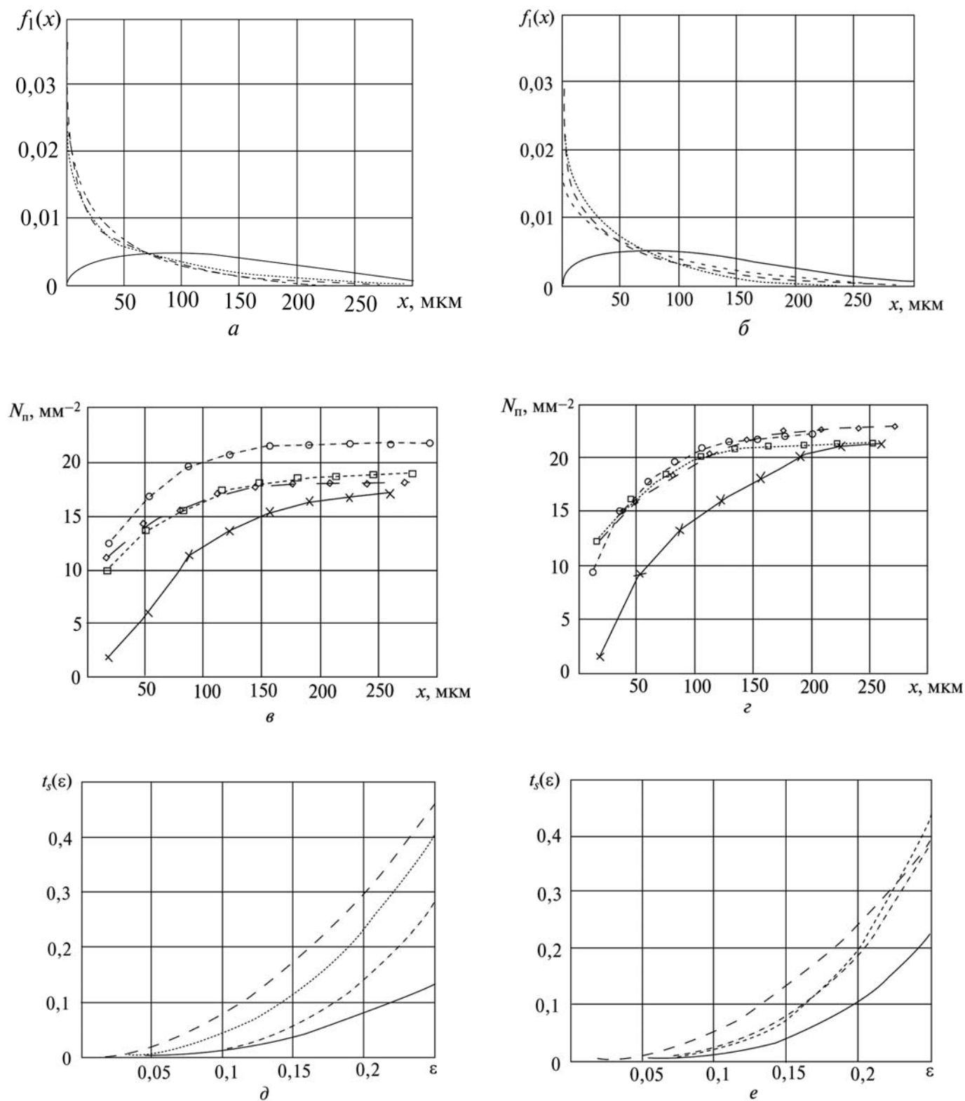
Рис. 3. Характеристики РП некоторых кругов:
