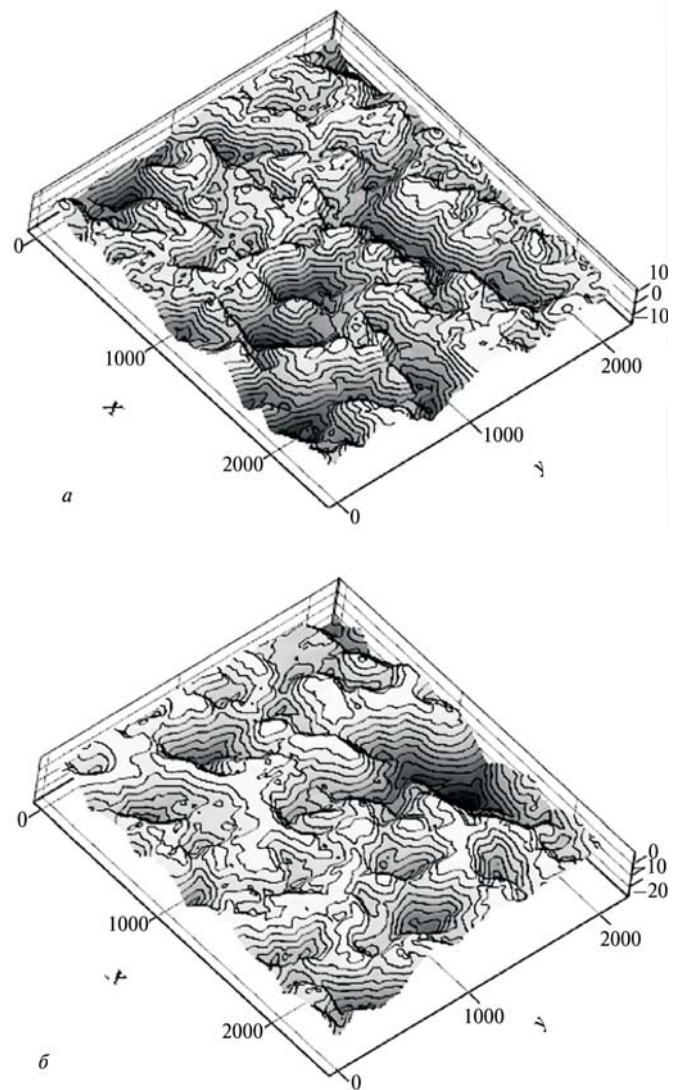
Рис. 2. Топограмма РП ШК ПП 125×16×32 25А 25-Н СМ2 7 К (WA F60 L 7 V):
