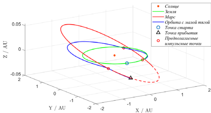
Рис. 7. Предполагаемые точки импульса на топливо-оптимальной орбите с малой тягой
