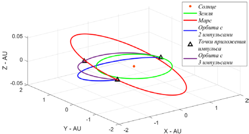
Рис. 3. Орбита трехимпульсного перелета
