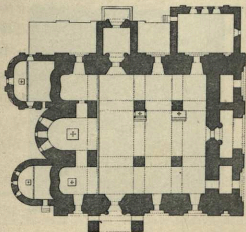
Архангельскій соборъ въ Москвѣ.
