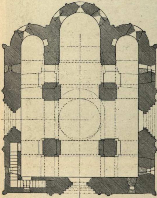
Планъ Успенскаго собора въ Звенигородѣ.
