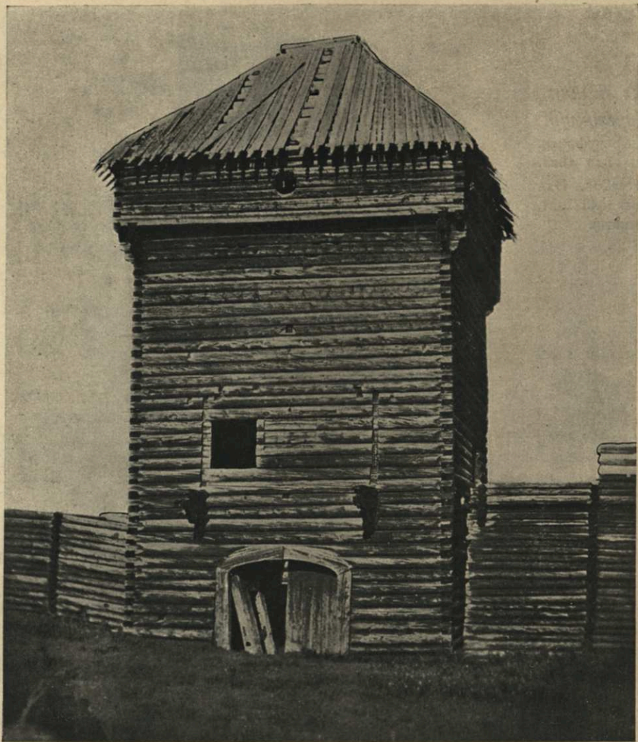
Главная башня Якутскаго острога—1683 г.
