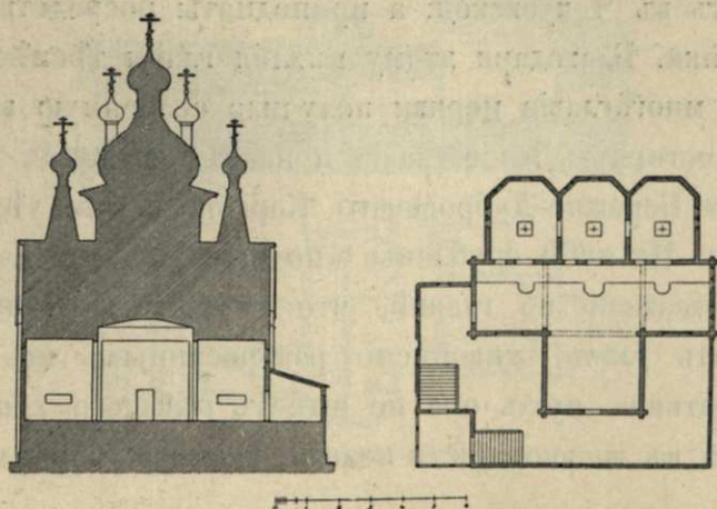
Церковь Владимірской Божіей Матери въ Подпорожьи Архангельск. губ. Онежск. уѣзда.—1745 г. (Фот. и обмѣры В. В. Суслова).
