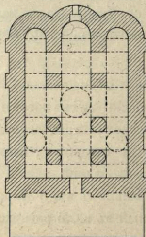
Церковь Іоанна Предтечи. — 1240 г. Западная сторона церкви и планъ ея. (Фот. Е. Ф. Елизарова въ Псковѣ).
