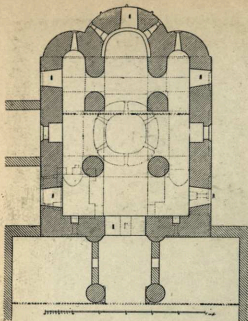
Планъ Дмитріевскаго собора въ Гдовѣ.—1540 г. (По объѣмамъ П. П. Покрышкина). 1540 г.
