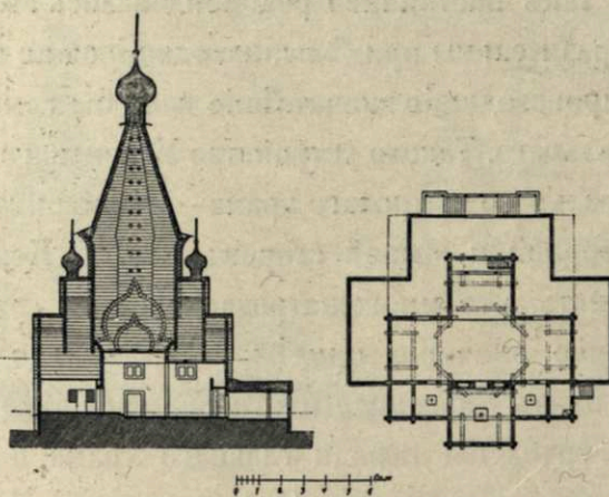
Климентовская церковь въ посадѣ Уга Архангельск. уѣзда. —16-й вѣкъ. (Фот. и обмѣры В. В. Суслова).
