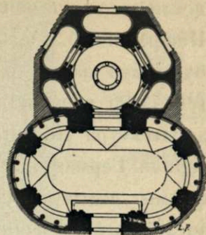
Santuario della Madonna della Consolata. (Туринъ).
