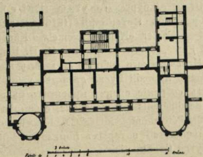
Луиджи Руска. Домъ Мятлева, нынѣ графовъ Бобринскихъ въ Спб.
