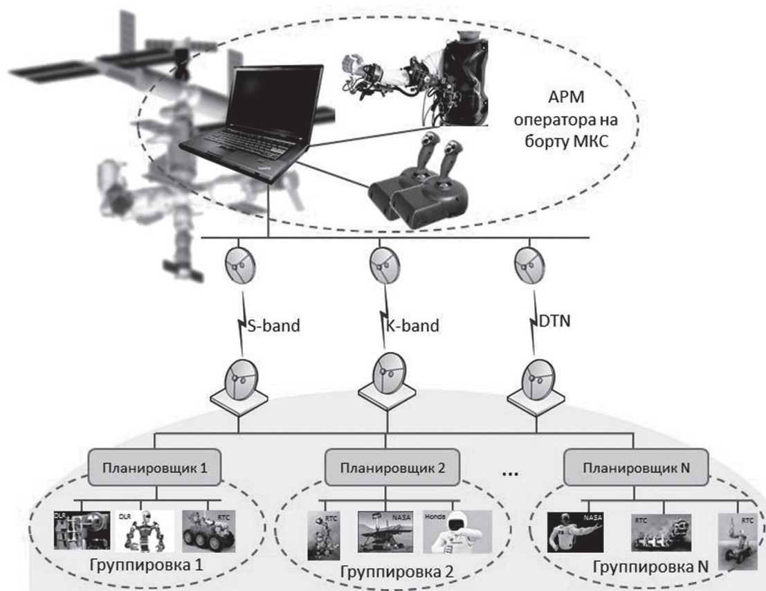
Рис. 3. Возможности управления напланетными автоматизированными устройствами Fig. 3. Opportunities of planetary automated control devices
