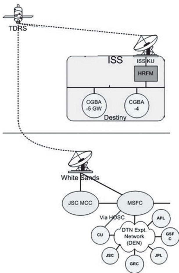
Рис. 2. Схема DTN-сети МКС Fig. 2. A scheme of a DTN network of ICS
