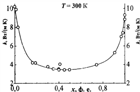
Рисунок 3. Концентрационная зависимость теплопроводности твердого раствора \text{Ca}_{1-x}\text{Sr}_x\text{F}_2
