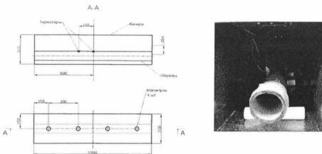
Рис. 7. Схема размещения заготовки детали внутри камеры СВЧ-нагрева
