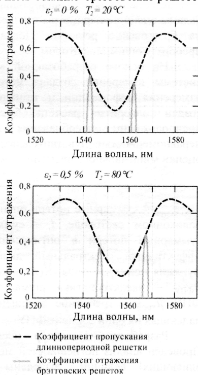
Рисунок 5. Спектр излучения, отраженного от гибридного много-решётчатого датчика
