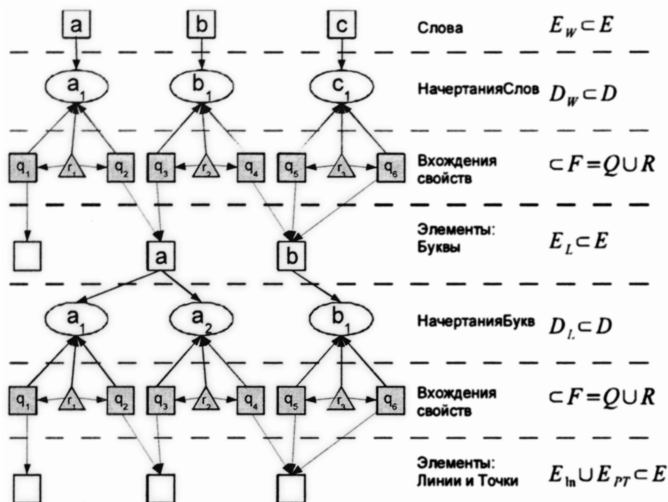
Рис.5. Схема построения базы знаний.
