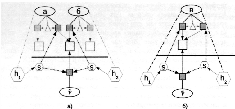
Рис. 6. Виртуальный фрейм и гипотезы (на рисунке: \tilde{v} - виртуальный фрейм; h_1, h_2 - узлы гипотез; s - узлы пар согласований из S(h) ).
