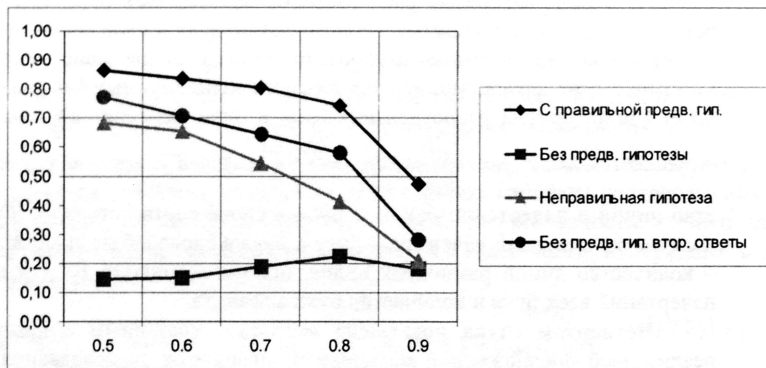
Рис. 7. Результаты исследования корректности алгоритма распознавания букв
