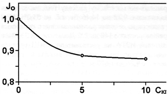
Рис. 9. Зависимость обобщенной целевой функции J_0 от содержания кукурузного масла в смеси C_{км}
