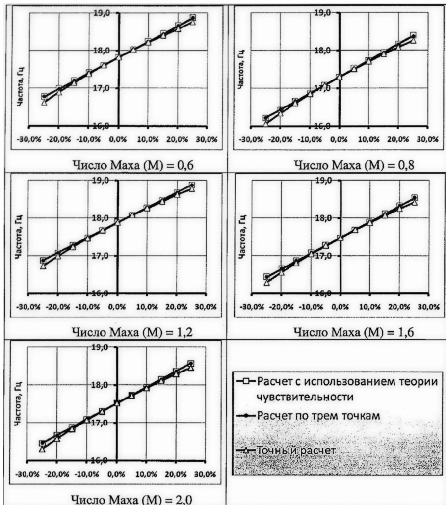
Рисунок 15. Изменение частоты 1-го тона в зависимости от вариации жесткости 1-й области пластины
