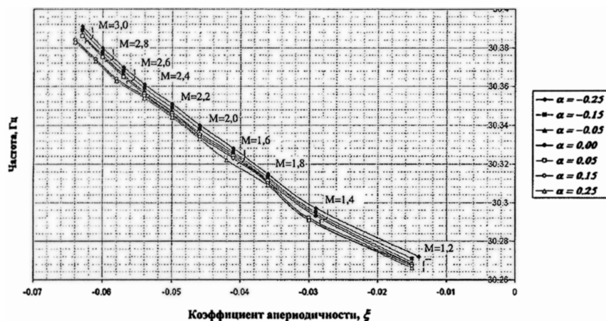
Рисунок 18. Изменение частоты колебаний 1-го тона ракеты в потоке в зависимости от вариации \alpha жесткости 2-й области конструкции (задних несущих поверхностей) и 5-й области конструкции (крепление задних несущих плоскостей) для разных чисел Маха
