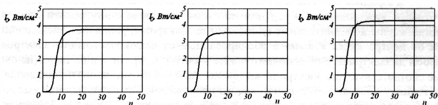
Рис. 9. Зависимости интенсивности оптического поля на оси от номера итерации при различных профилях распределения усиления
