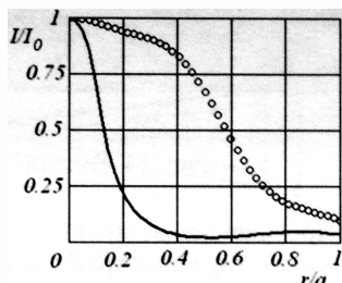
Рис. 12. Радиальные распределения интенсивности индуцированного излучения
