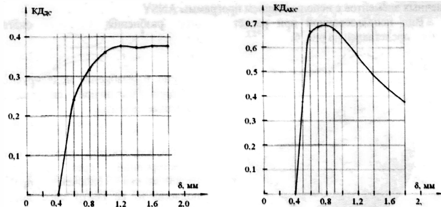
Рис. 4. Зависимости критериев добротности датчика силы KD_D и акселерометра KD_{AKC} от величины рабочего зазора \delta датчика силы.
