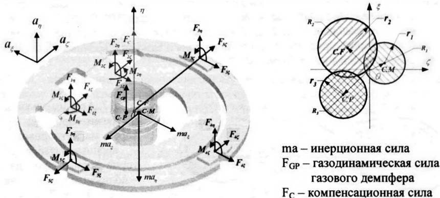
Рис. 5. Схема нагружения маятникового узла акселерометра.
