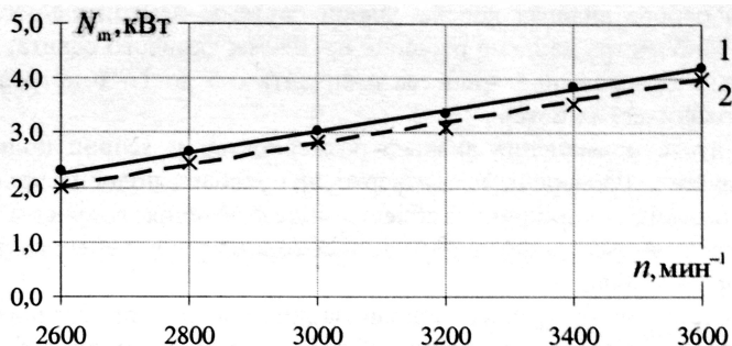
Рис.7. Характеристики общих механических потерь дизеля ТМЗ-450Д при использовании обычного (1) и энергосберегающего (2) моторного масла
