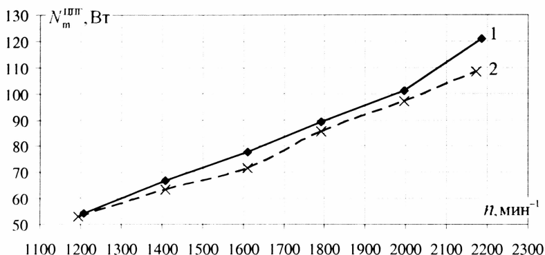
Рис.6. Вид и сопоставление экспериментальных характеристик механических потерь в ЦПГ поршневого трибометра при смазывании обычным (1) и энергосберегающим (2) моторными маслами температурой 70°C
