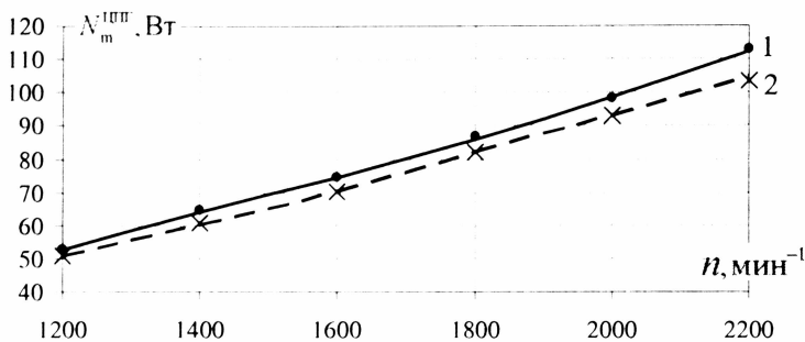
Рис.3. Расчетная характеристика механических потерь в ЦПГ поршневого трибометра при использовании различных моторных масел: 1 - обычное; 2 - энергосберегающее
