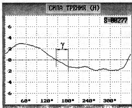
Рис.1. Расчетное (а) и экспериментальное (б) проявление фазового сдвига \gamma нулевого значения силы трения в окрестности мертвых точек
