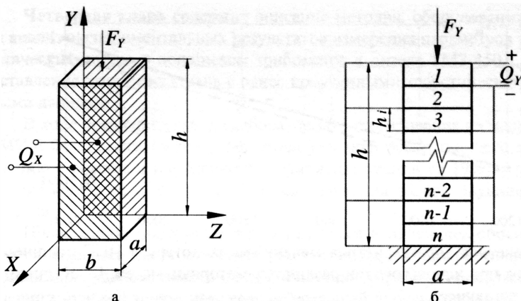
Рис.2. Расчетная схема и структура однослойного поперечного (а) и многослойного продольного (б) пьезоэлементов датчика силы трения
