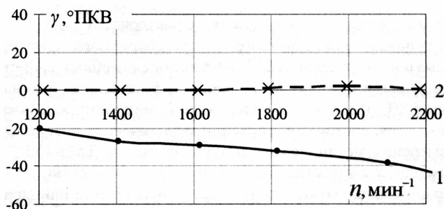
Рис.5. Значение угла фазового сдвига нулевой точки силы трения на измерительной полосе поршневого трибометра в зависимости от скоростного режима до (1) и после (2) модернизации измерительного узла
