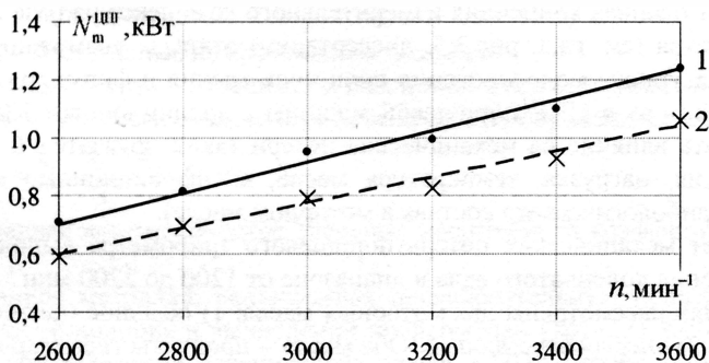
Рис.4. Расчетная характеристика механических потерь в ЦПГ дизеля ТМЗ-450Д при использовании различных моторных масел: 1 - обычное; 2 - энергосберегающее
