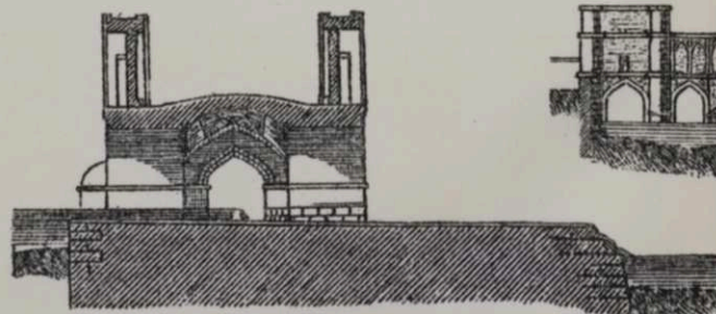
Чер. 182 б.
