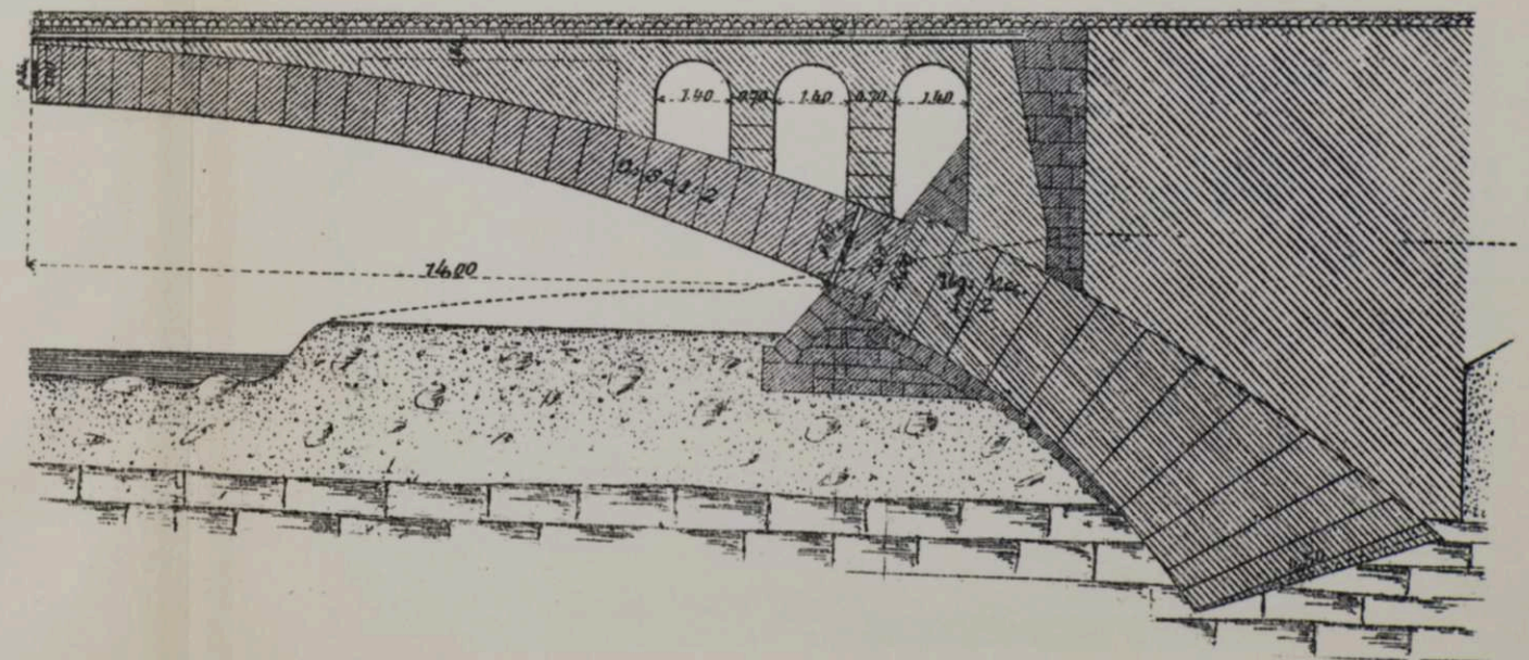
Чер. 326. Мостъ чер. Enz бл. Hofen.
