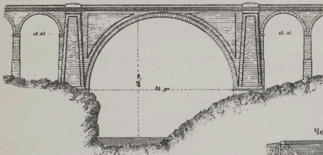
Чер. 294. Мостъ въ Tilsit.
