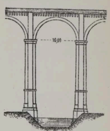
Чер. 251. Виадукъ Dinan.
