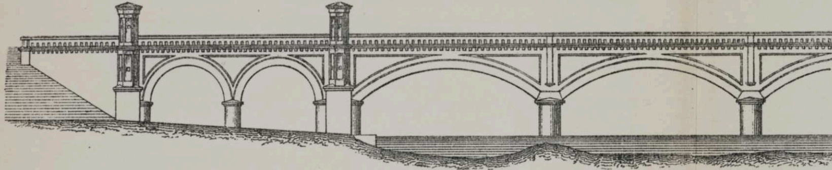
Чер. 324 а.
