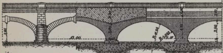
Чер. 286.01 Чер. 286. Мостъ Nogent.
