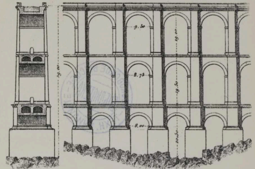
Чер. А Виадукъ Albano-Ariscia.
