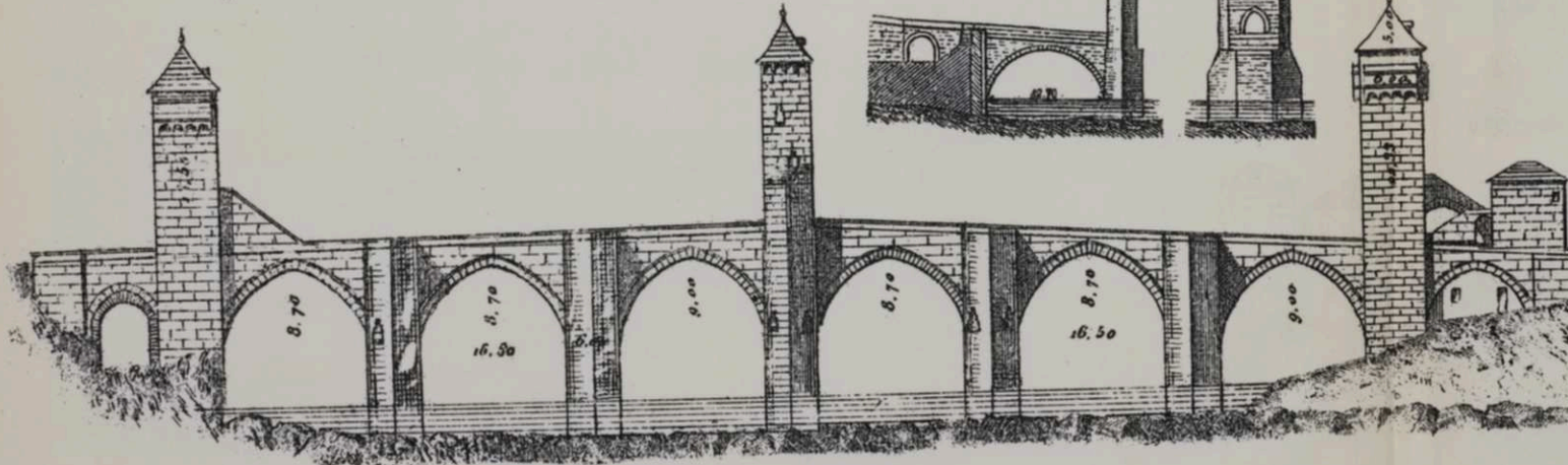
Чер. 118. Мостъ Valentré (de la Calendre).
