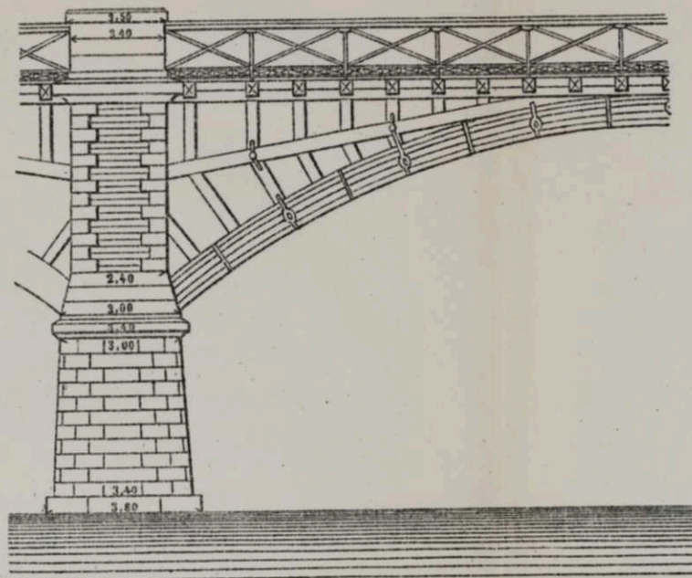
31. Мостъ въ Montlouis на Лоарѣ (проектъ).
