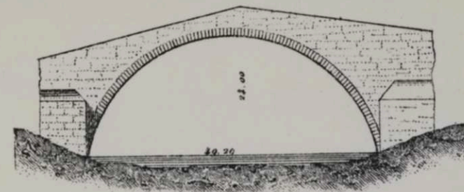
Чер. 141 а
