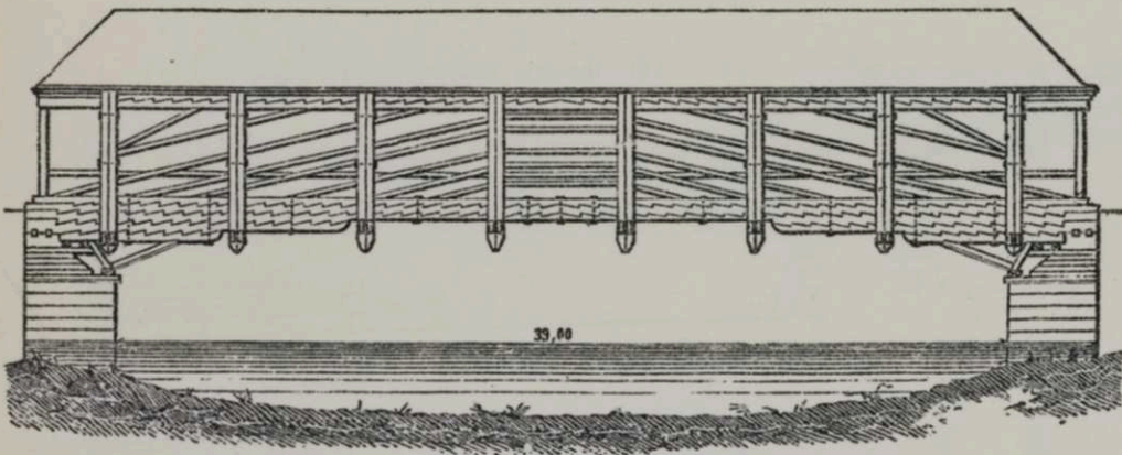
22. Мостъ черезъ Limmat близъ Wettingen (1778).
