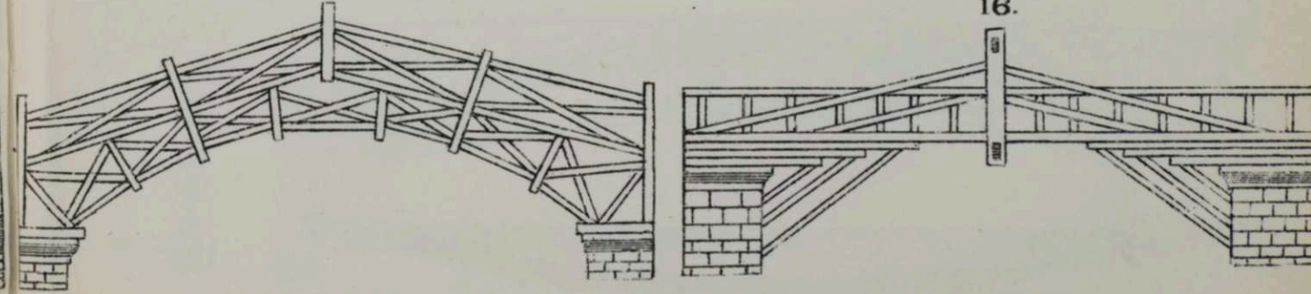
15. Ферма Fayolle (18 ст.)
