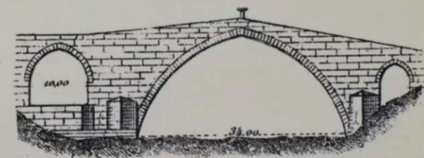
Чер. 124. Мостъ въ Козенъ чер. Saale.
