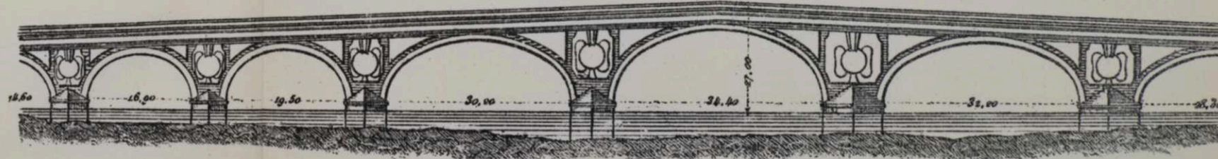
Чер. 166. Мостъ въ Тулузѣ чер. Гаронну.
