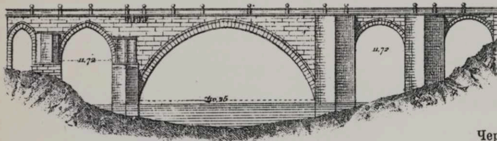
Чер. 114. Мостъ St. Martin чер. Тажъ.
