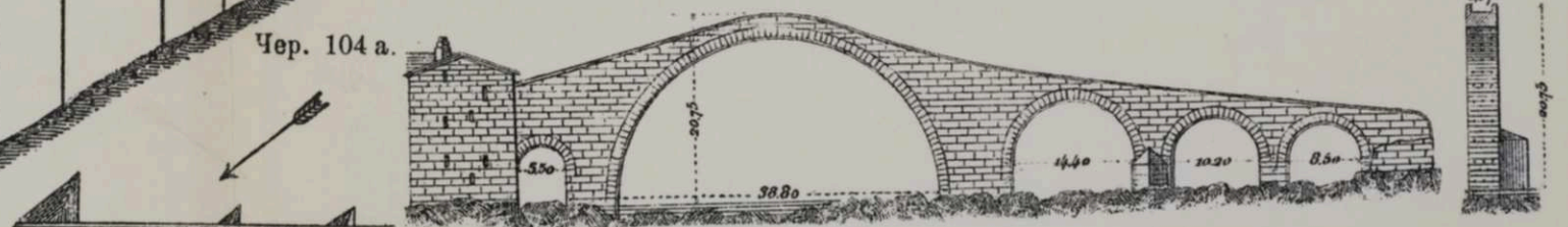
Чер. 98. Акведукъ Бургасъ.
