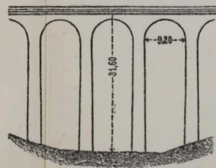
Чер. 270. Виадукъ Folkestone.
