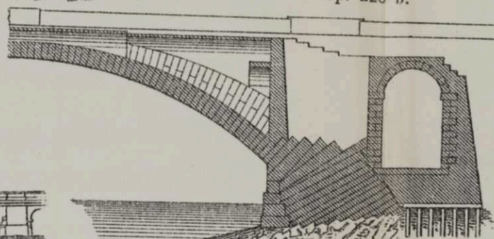
Чер. 228 б.
