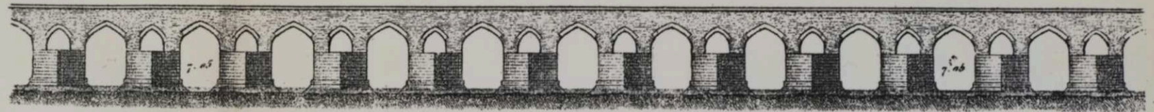
Чер. 179. Дѣвичій мостъ (Доктаре Поль).
