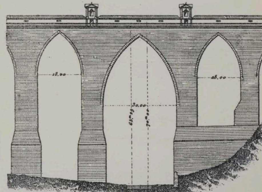
Чер. 223. Акведукъ Cysylltau.
