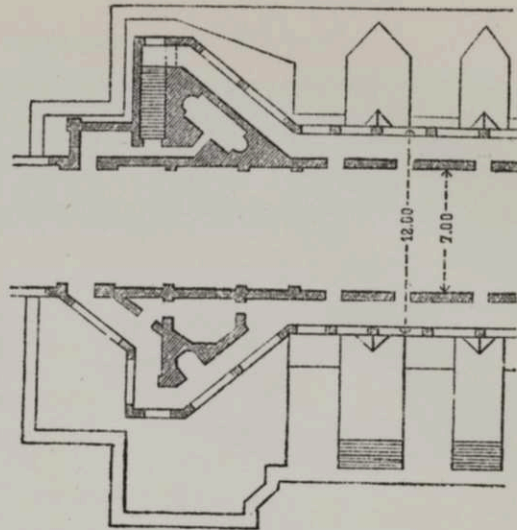
Чер. 183 д.
