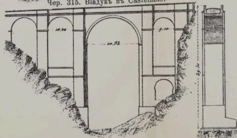
Чер. 315. Виадукъ въ Castellano.
