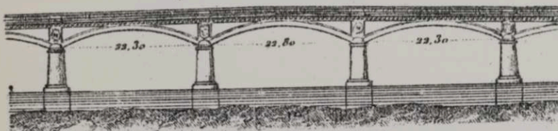
Чер. 297. Мостъ Port Sainte-Marie.
