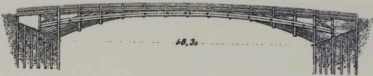
24. Мостъ въ Шердингъ (Баварія).
