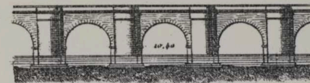
Чер. 215. Мостъ Mançanages.
