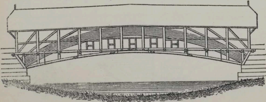
23 Мостъ черезъ Reuss въ Mellingen.
