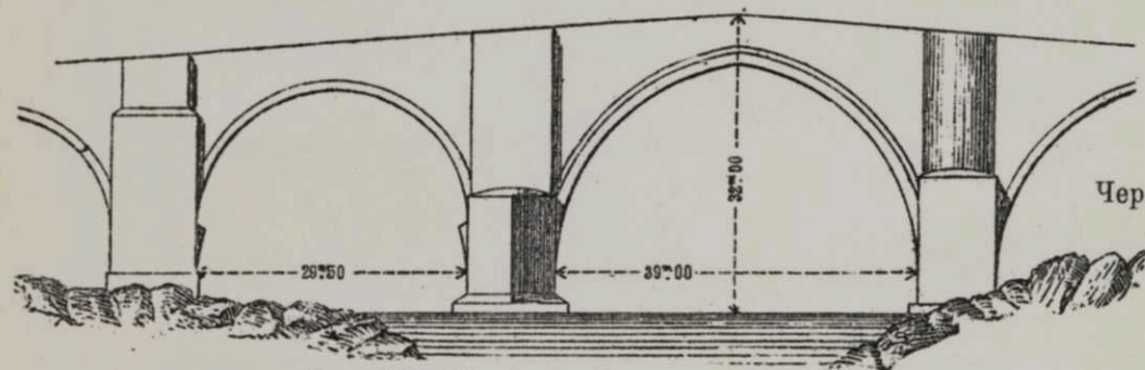
Чер. 131. Мостъ въ Seret чер. Tech.
