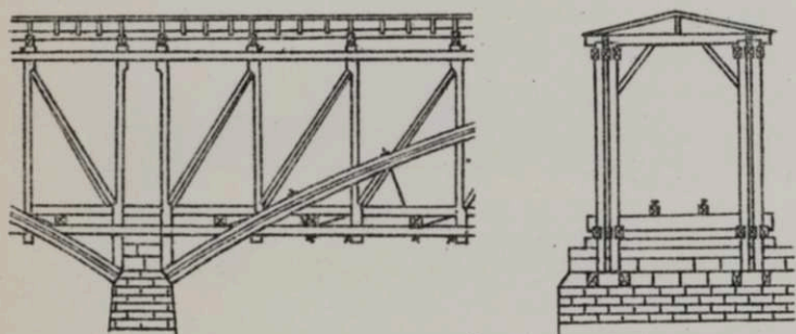
37. Система Лонгъ.
