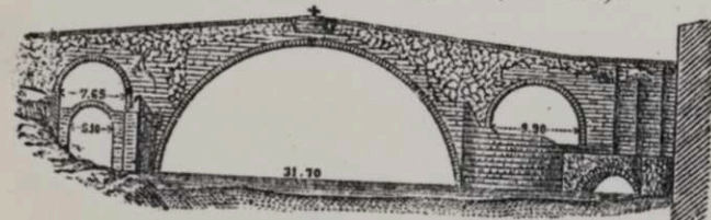
Чер. 134. Мостъ Olargues (Hérault).
