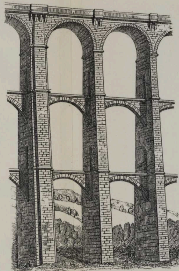
Чер. 253 б.
