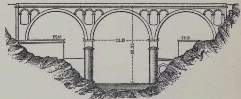
Чер. 271. Виадукъ Linlithgow.
