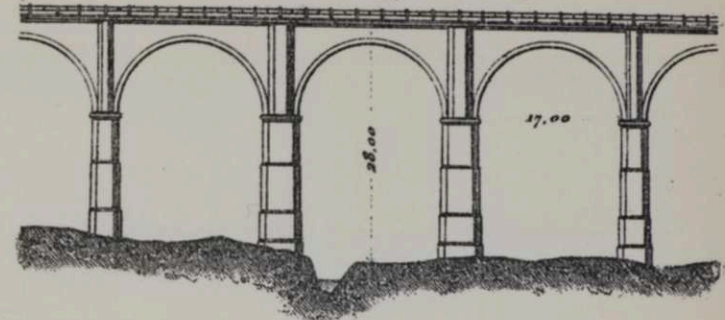
Чер. 264. Виадукъ Löbau.
