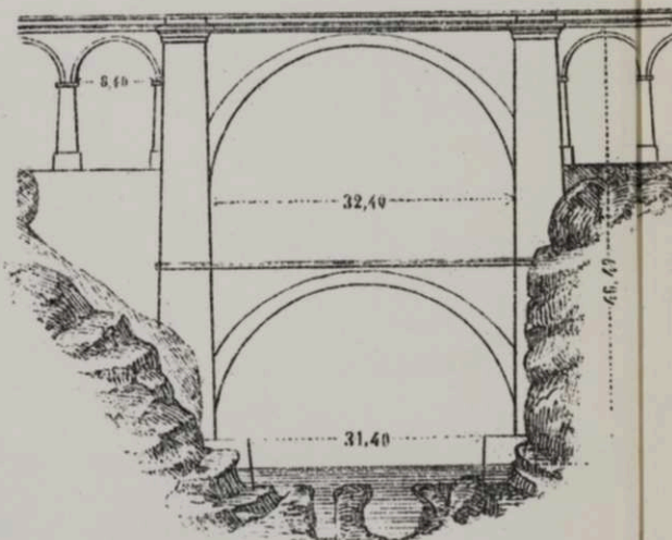
Чер. 258. Виадукъ Port Launey.
