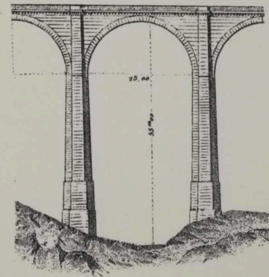
Чер. Р Виадукъ Помпадуръ.
