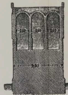
Чер. 179 б.
