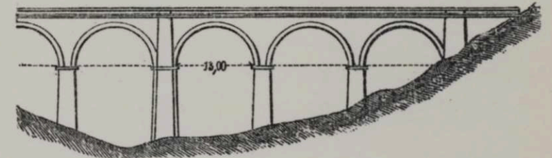
Чер. 321. Мостъ чер Garganta Ancha.
