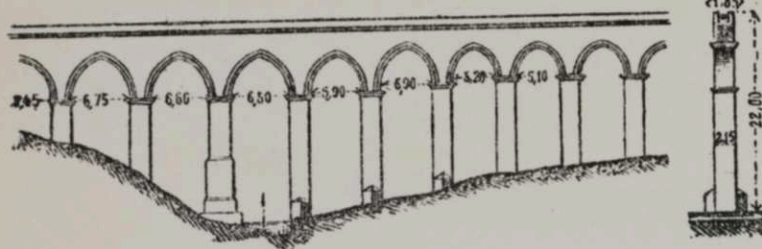
Чер. 149. Мостъ Carodars въ Сициліи.
