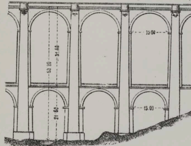
Чер. 256. Виадукъ Altier.
