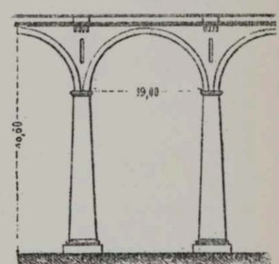
Чер. 254. Виадукъ Commelle.
