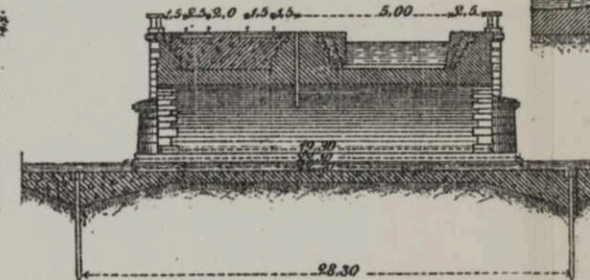
Чер. 289. Мостъ St. Sauveur.
