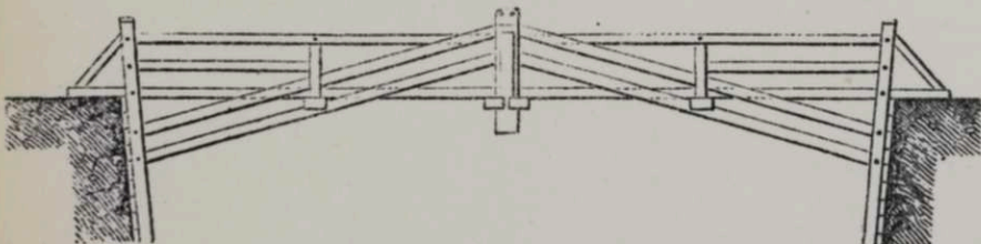
6. Мостъ въ Utrecht (Палладіо, 1518—1560)
