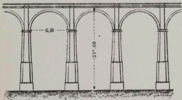
Чер. 259. Виадукъ Morlaix.
