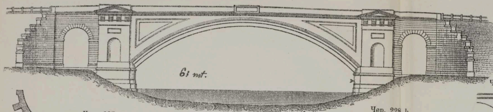
Чер. 228 а.
