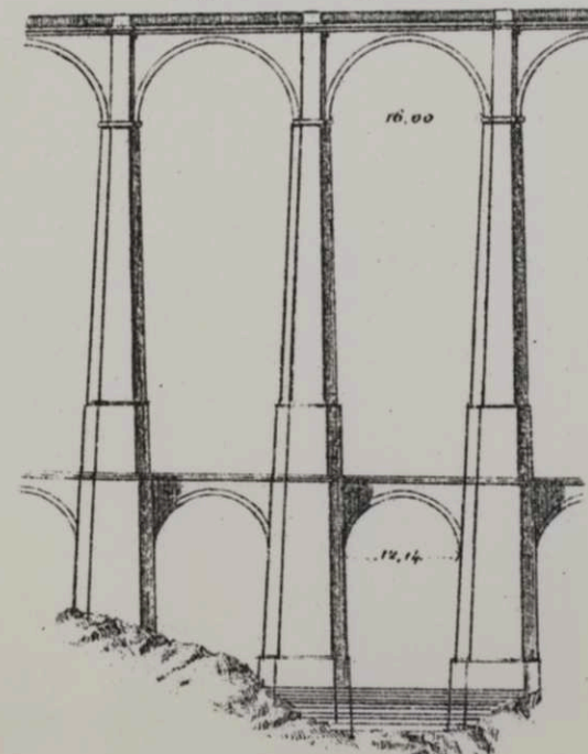
Чер. 256. Виадукъ Altier.
