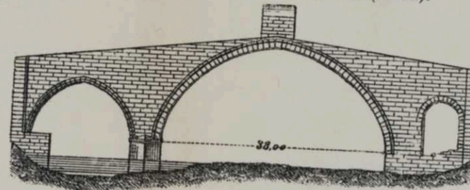
Чер. 105. Мостъ Martorelle (Нова).
