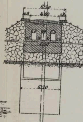
Чер. 324 а.
