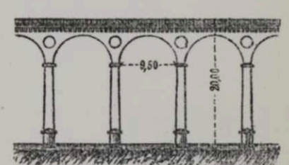
Чер. 257. Виадукъ Chatellux.
