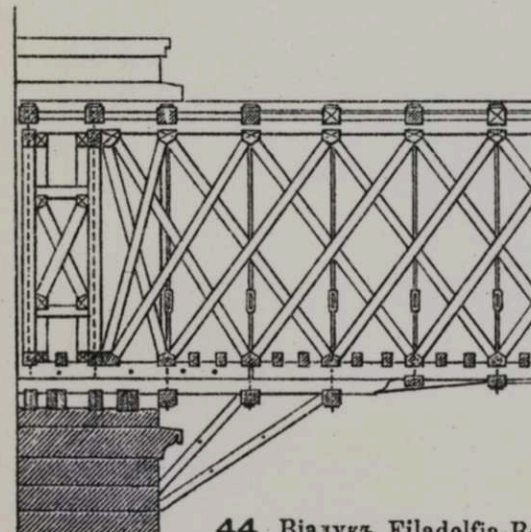
44. Виадукъ Filadelfia-Reading.
