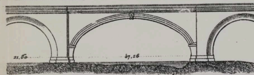
Чер. 206. Мостъ въ Lavour.
