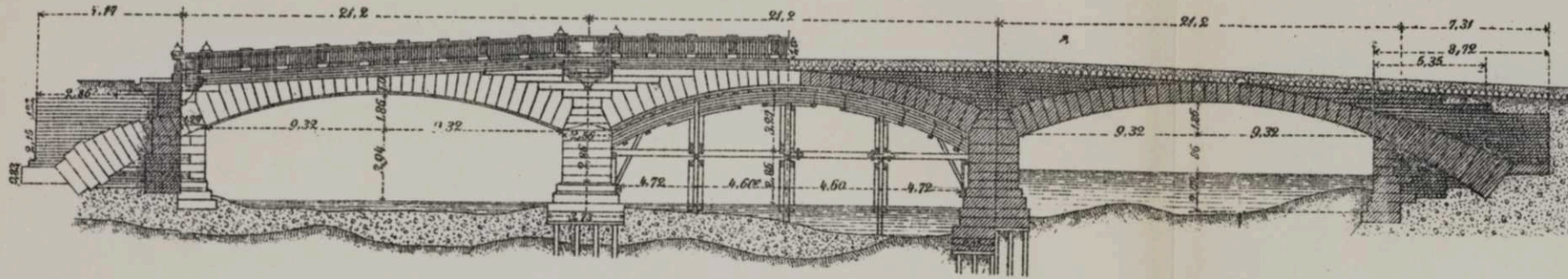
Чер. 318. Мостъ чер. Warthe бл. Wronke.
