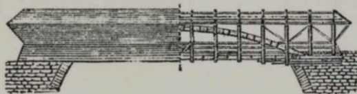
21. Мостъ въ Шафраузенъ на Рейнѣ (1757).
