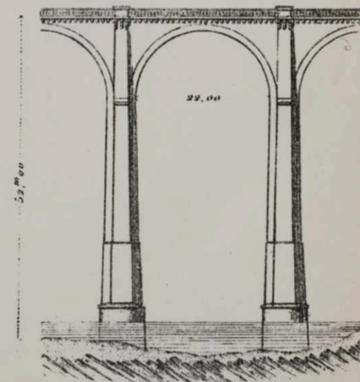
Чер. 258. Виадукъ Port Launey.
