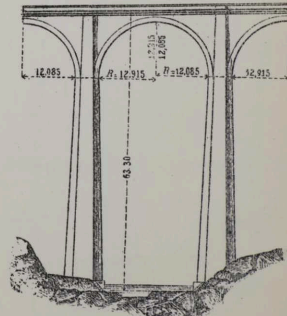
Чер. 260. Виадукъ Gruize.
