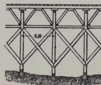
44. Виадукъ Filadelfia-Reading.
