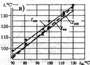
Рис. 27. а), б) – зависимость приращения температуры вкладышей от частоты вращения и от давления масла; в) – зависимость температуры вкладышей от температуры масла; t_{шв} , t_{шн} , t_{кн} – температура соответственно шатунного верхнего, нижнего и коренного вкладыша
