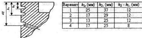
Рис. 11. Расположение канавок под компрессионные кольца
