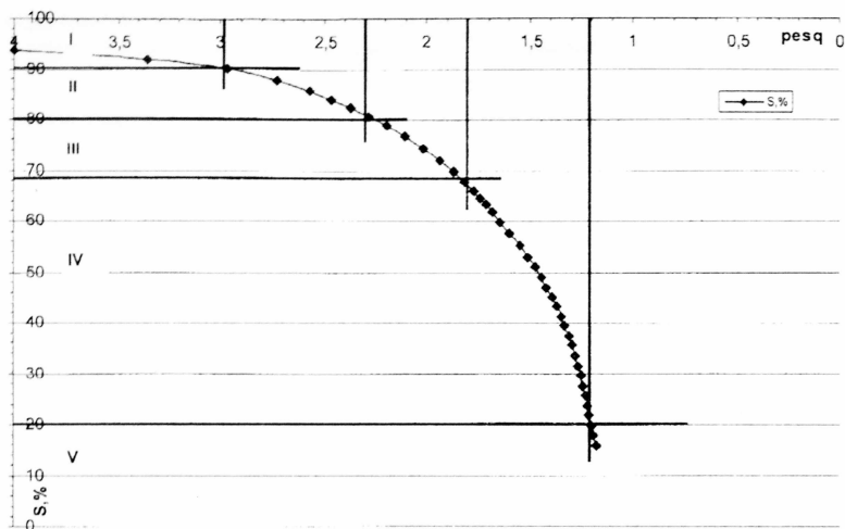
Рис. 2. Зависимость между значением автоматической оценки качества речи PESQ и слоговой разборчивости
