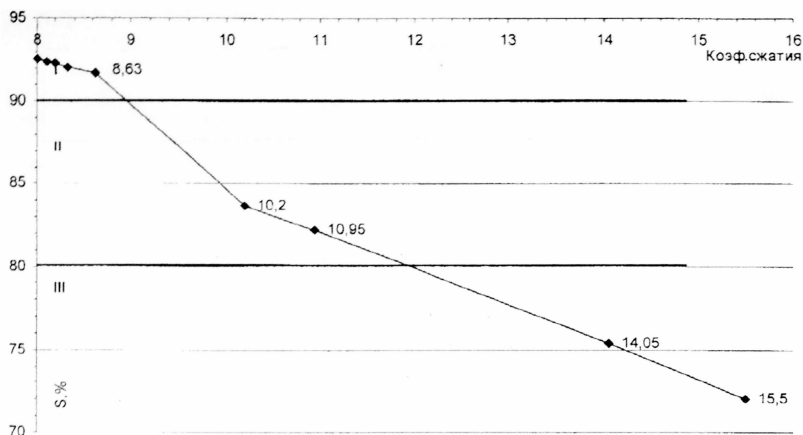
Рис. 3. Зависимость разборчивости восстановленной речи от коэффициента сжатия кода
