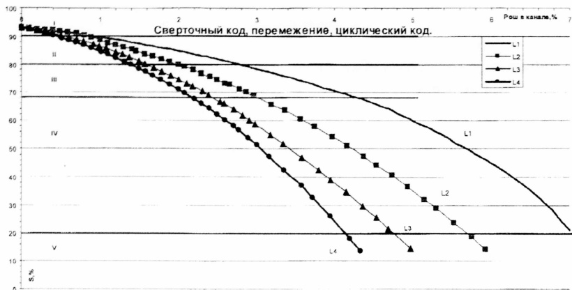
Рис. 8. Зависимость слоговой разборчивости от вероятности ошибки в канале связи стандарта GSM
