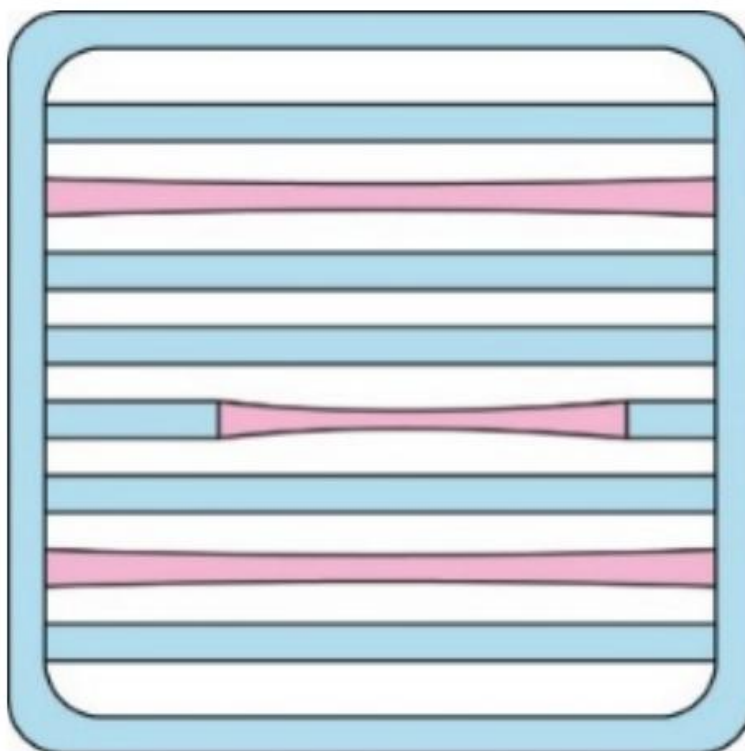
Рис. 3. Дефект недостаточной экструзии
