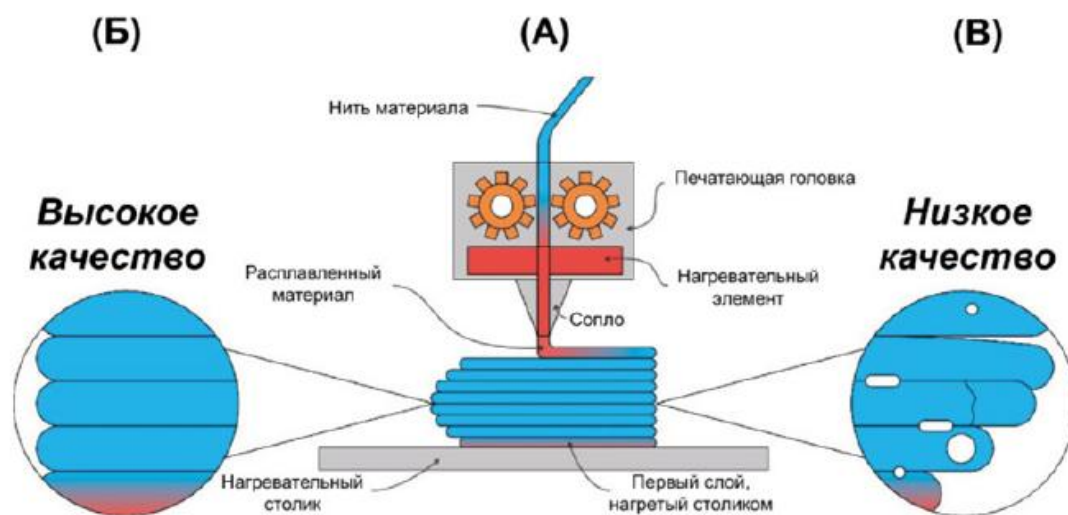
Рис. 1. Схема метода FDM:
