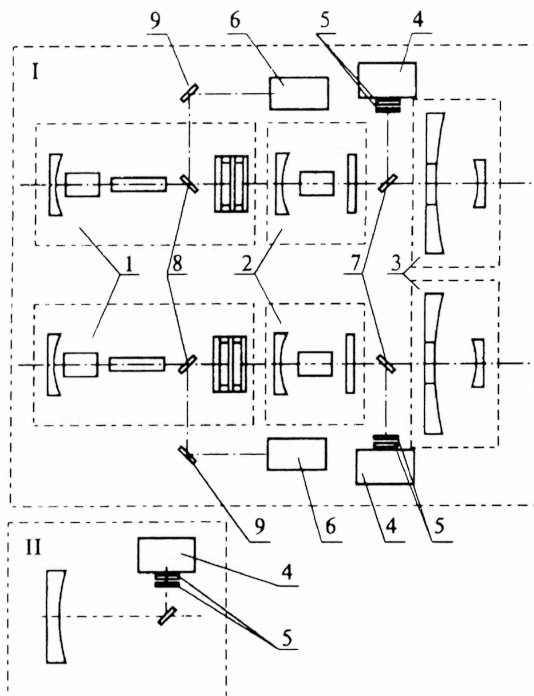
Рис. 12. Функциональная оптическая схема лидара
