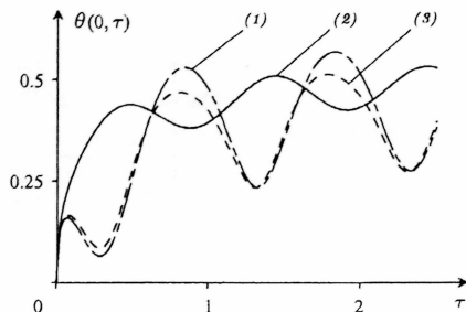
Рис. 5. Температура границы x = 0 полупространства при реализации различных режимов теплообмена с внешней средой и различных законах движения покрытия:
