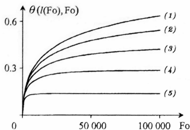
Рис. 4. Влияние скорости V_0 движения покрытия на температуру границы \xi = l(Fo) полупространства при A = 0.02 , B = 50 , D = 0.01 :
