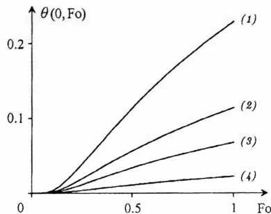
Рис. 2. Временная зависимость температуры контактной границы \xi = 0 при различных значениях параметра H :
