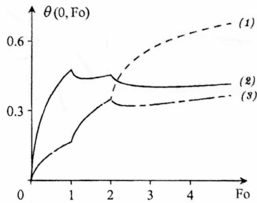
Рис. 3. Зависимость температуры границы \xi = 0 полупространства от числа Фурье Fo в импульсном режиме теплообмена с внешней средой при N = 2 , \gamma = 5 и различных значениях параметров \beta_0 , \beta_1 , \beta_2 : \beta_0 = 1 , \beta_1 = 2 , \beta_2 = 4 (1); \beta_0 = 4 , \beta_1 = 2 , \beta_2 = 1 (2); \beta_0 = 1 , \beta_1 = 2 , \beta_2 = 1 (3)
