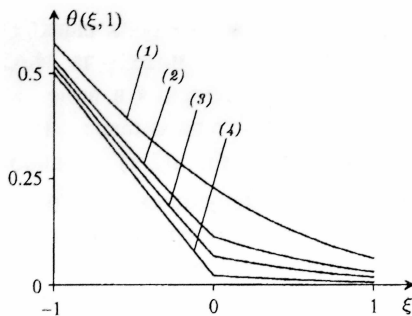
Рис. 1. Температурный профиль в системе “полупространство–теплозащитное покрытие” при различных значениях параметра H :
