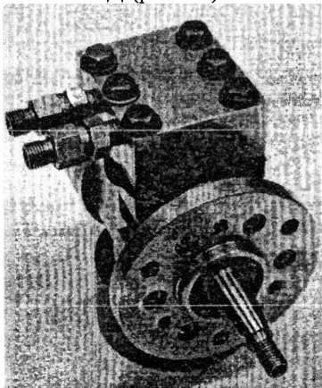
Рис. 12. Экспериментальный ТНВД для топливной системы CR.
