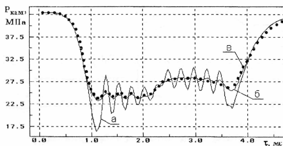
Рис. 5. Давление в камере управления ЭГФ БашГАУ: а – расчет без учета силы гидродинамического сопротивления, б – расчет с учетом силы гидродинамического сопротивления, в – эксперимент.
