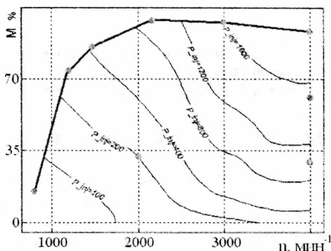
Рис. 11. Оптимальные значения давления впрыскивания в поле режимов дизеля ЗМЗ-514.
