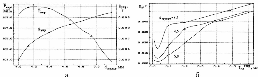
Рис. 4. Влияние мультипликатора записания на показатели ЭГФ с дроссельным управлением: а – среднее давление впрыскивания и цикловая порция топлива на управление; б – характеристика подачи в функции времени управляющего импульса.
