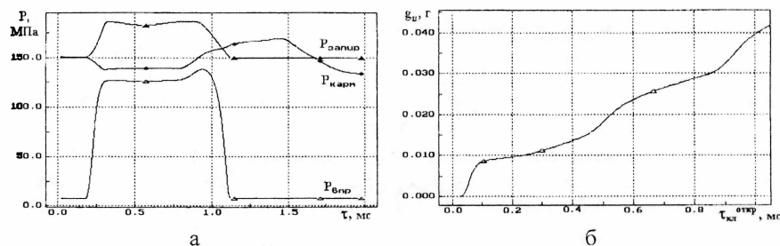
Рис. 3. Результаты численного исследования ЭМФ с замкнутой камерой над разгружающим плунжером при d_{пл}=3,65 мм, V_{кам}=105 мм 3 : а – мгновенные давления запирания, в кармане распылителя и впрыскивания; б – характеристика подачи в функции времени управляющего клапаном импульса.
