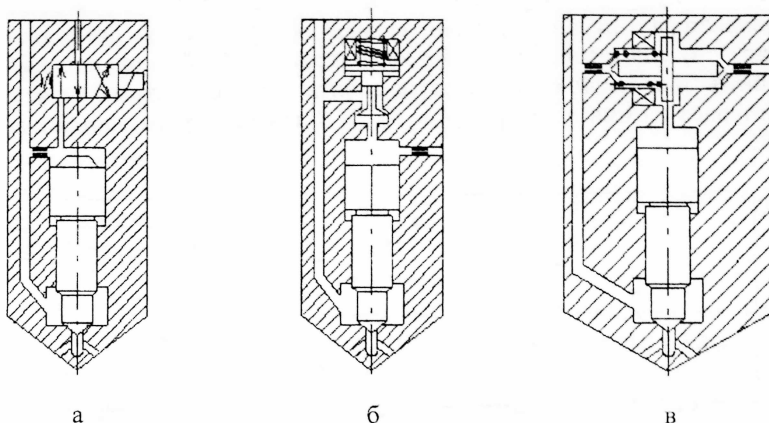
Рис. 2. Схемы ЭГФ: а – с золотником, б – с гидравлически разгруженным клапаном, в – с двухзатворным гидравлически разгруженным клапаном.
