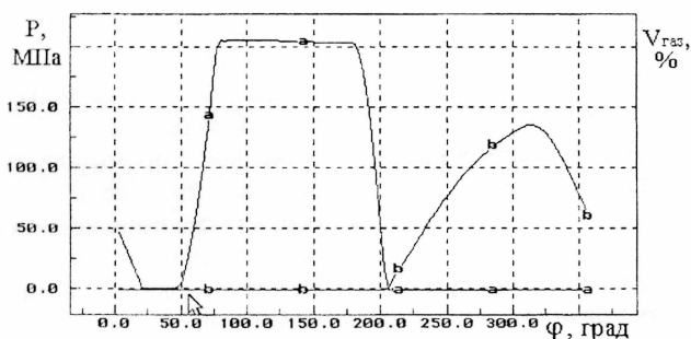
Рис. 10. Мгновенная величина давления (а) и газосодержания (б) в надплунжерной полости ТНВД в функции угла поворота приводного вала ТНВД.
