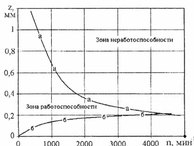
Рис. 9. Кривая работоспособности (а) для грибкового клапана диаметром 5 мм, массой 2,5 г; минимально необходимый подъем клапана (б).
