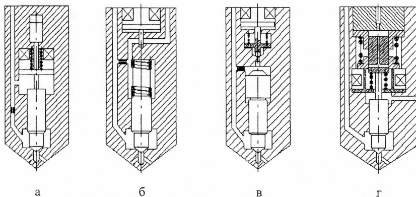
Рис. 1. Схемы форсунок: а – ЭМФ с замкнутой надплунжерной камерой, б – ЭГФ с дроссельным управлением, в – ЭГФ с мультипликатором запирания и отрицательной обратной связью по подъему иглы, г – ЭГФ со следящей системой привода иглы.
