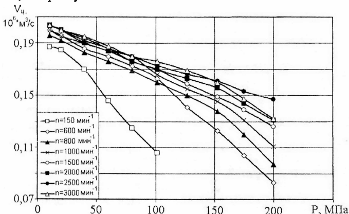
Рис. 13. Гидравлическая характеристика ТНВД МГТУ им. Н.Э. Баумана.
