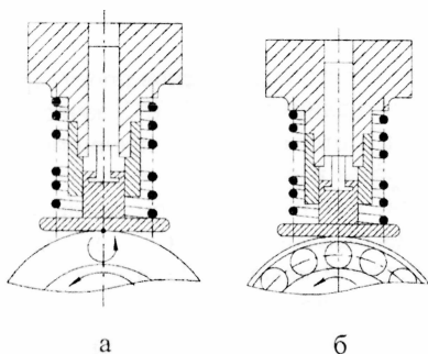
Рис. 7. Схемы приводов плунжеров: а – с подшипником скольжения, б – с иглольчатым подшипником.
