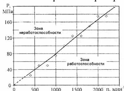
Рис. 8. Кривая работоспособности подшипника скольжения.
