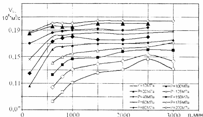
Рис. 14. Зависимость объемной цикловой производительности ТНВД МГТУ им. Н.Э. Баумана от частоты вращения его вала при различных давлениях подачи.
