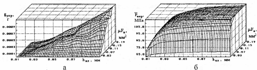
Рис. 6. Влияние хода двухзатворного клапана и последовательно установленных жиклеров ЭГФ с двухзатворным гидравлически разгруженным клапаном: а – цикловая порция топлива на управление; б – среднее давление впрыскивания в функции.
