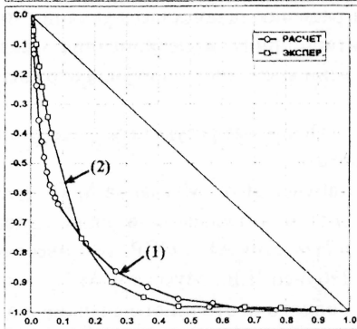
Рис. 15. Распределение нормированной ЭПР самолета МИГ-23 в горизонтальной плоскости: (1) - расчет; (2) - эксперимент.
