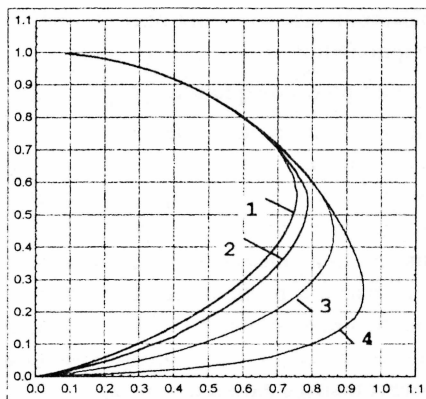
Рис. 3. Индикатрисы вероятности q_{\infty}(0, \tilde{y}_0 | \alpha) не затенения луча:
