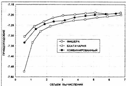
Рис. 1. Функционалы качества обучения SVM алгоритма.
