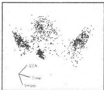
Рис. 11. Кластеры объектов.
