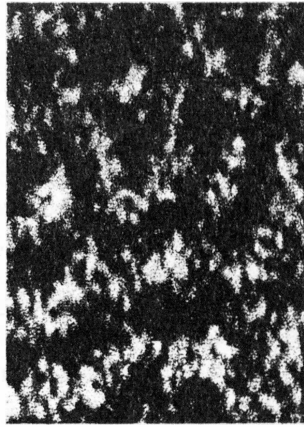
Рис. 4. Радио-изображение моря.
