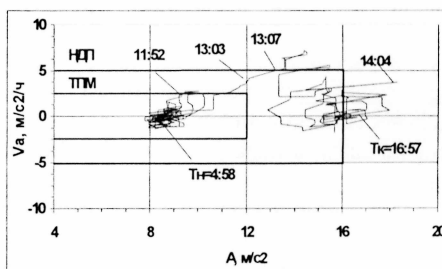
Рис. 8. Диагностика и прогнозирование состояния насосного агрегата: а) прогноз разрушения подшипника по трендам виброускорения A(t) и скорости его роста Va(t) ; б) диагностика на фазовой плоскости A - Va
