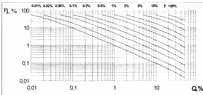
Рис. 1. Допустимая ошибка системы мониторинга \eta при требуемом риске r пропуска отказа и фактической вероятности отказа НХК – Q
