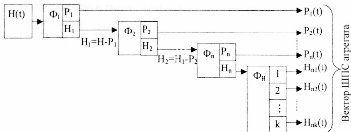
Рис. 2. Алгоритм рекуррентной фильтрации ШПС как функций времени:
