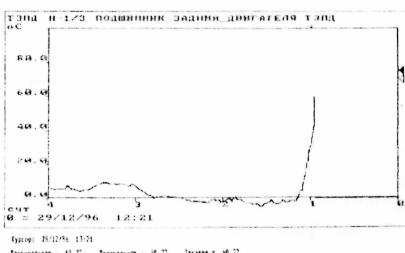
Рис. 7. Быстрые тренды диагностических сигналов: а) виброперемещения при ослаблении крепления насоса НК210; б) температуры подшипника скольжения электродвигателя ВАО500L-2 центробежного насосного агрегата НПС200/700
