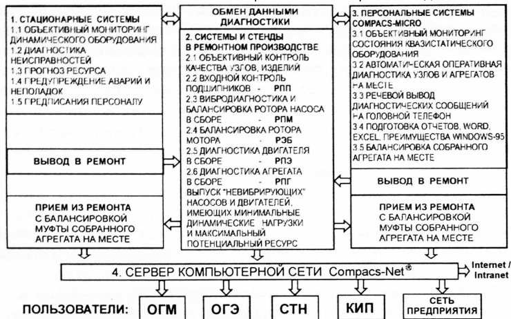
Рис. 11. Автоматизированная система управления и технология безопасной ресурсосберегающей эксплуатации агрегатов НХК:
