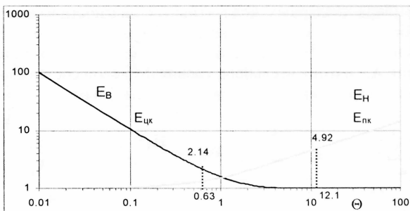
Рис. 5. Эффективность метода синхронной пиковой демодуляции
