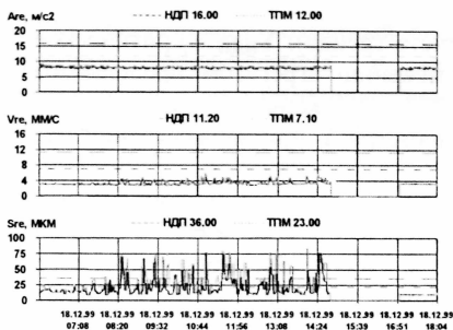
Рис. 6. Вибрация двигателя ВАО-71-292 при ослаблении крепления: а) тренды A , V , S до и после ремонта; б) спектры V , S перед ремонтом
