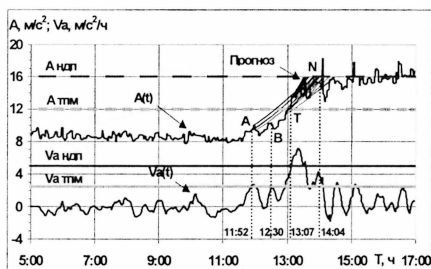
Рис. 8. Диагностика и прогнозирование состояния насосного агрегата: а) прогноз разрушения подшипника по трендам виброускорения A(t) и скорости его роста Va(t) ; б) диагностика на фазовой плоскости A - Va
