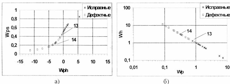
Рис. 4. Разделение агрегатов на два класса с исправными и дефектными подшипниками качения в координатах диагностических признаков:
