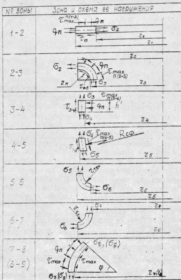
Рис. 4. Зоны очага деформации при фрикционно-реверсивной вытяжке эластичным пусковым по жесткой матрице и схеме напряжений, действующих на каждую из нит.
