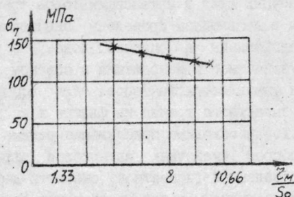
Рис. 5.2. Зависимость меридионального напряжения в опасном сечении от относительного радиуса закругления рабочей кромки матрицы.
