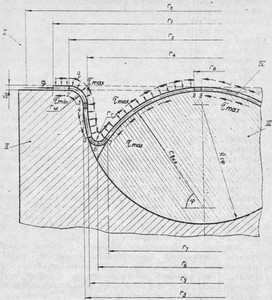
Рис.3. Структурная схема для анализа напряженно-деформированного состояния заготовки при фрикционно-реверсивной вытяжке эластичным пуансоном по жесткой матрице:
