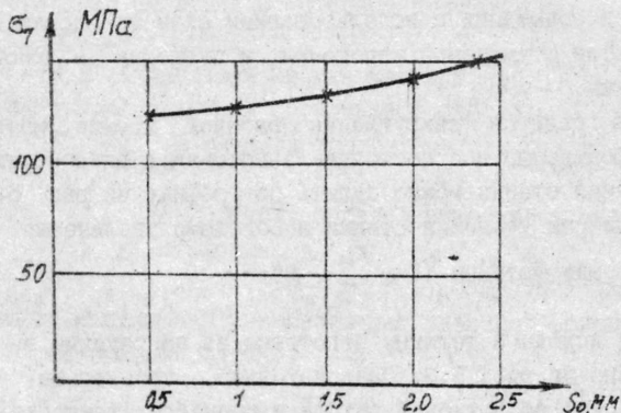
Рис. 5.3. Зависимость меридионального напряжения в опасном сечении от исходной толщины заготовки.
