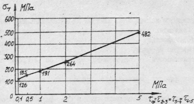
Рис. 5.1. Зависимость меридионального напряжения в опасном сечении от напряжений контактного трения.
