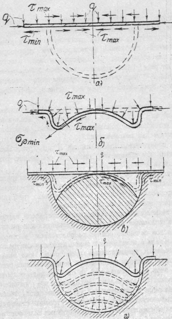
Рис. I. Структура формирования и технологическая схема процесса фрикционно-реверсивной вытяжки эластичной среды по жесткой матрице:
