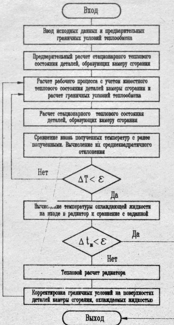
Рис.1. Блок-схема теплового расчета СО дизеля
