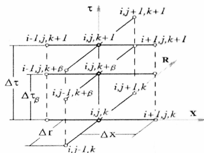
Рис. 3. Шаблон схемы расчета
