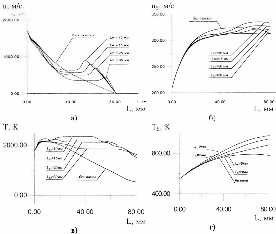
Рис. 4. Распределение осевой скорости и температуры для различных L_m и без маски ( d_s=30 мкм, Z=10\% , D_m=7 мм, 2\alpha_m=90^\circ , L_n=80 мм)
