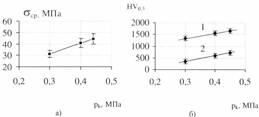
Рис. 5. Зависимость адгезионной прочности и твердости от давления в КС
