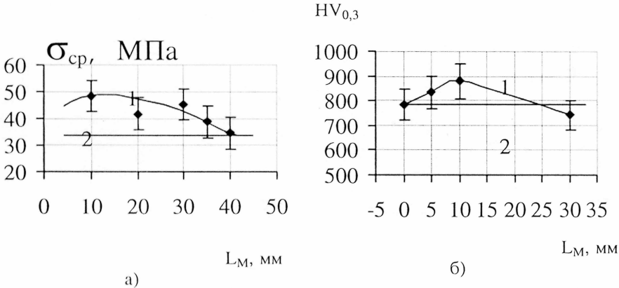
Рис. 7. Зависимость адгезионной прочности и твердости от расстояния между выходным сечением насадка и передней кромкой маски
