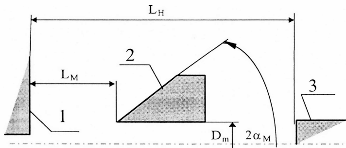
Рис. 1. Схема установки: 1 — выходное сечение насадка установки СГН; 2 — сепарирующее устройство (маска); 3 — напыляемый цилиндрический образец
