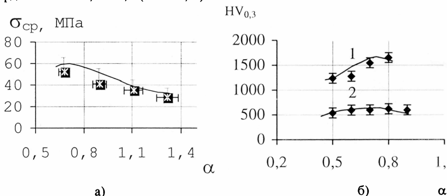
Рис. 6. Зависимость адгезионной прочности и твердости от коэффициента избытка окислителя
