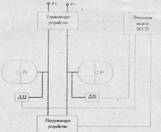
Рис.1. Общая схема имитаторов гидропривода.
