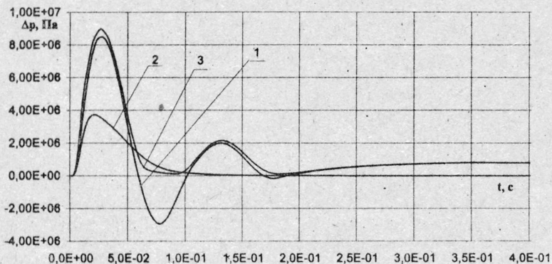
Рис.2. Переходный процесс по перепаду давлений.
