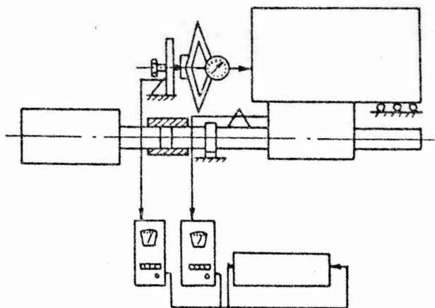
Схема замера жёсткости
